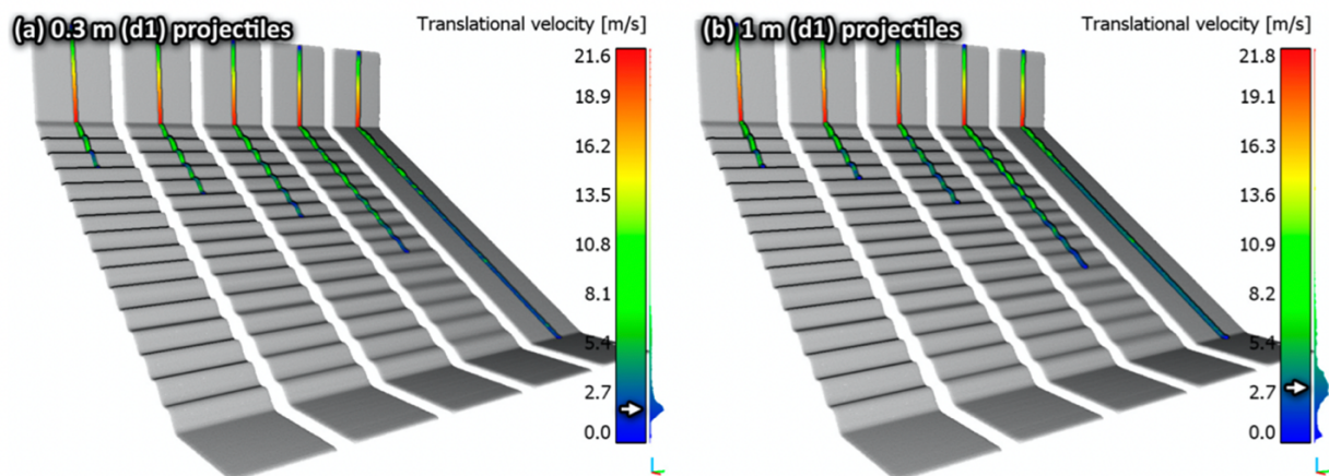
Figur 73: Senterlinja til simulerte steinsprangutløp til blokker med ulik størrelse. Hastigheita til blokkene, vist med farge, aukar med auka blokkstorleik. Utløpslengda avheng av hastigheita og ruheita til terrenget (Noël et al., 2021).
