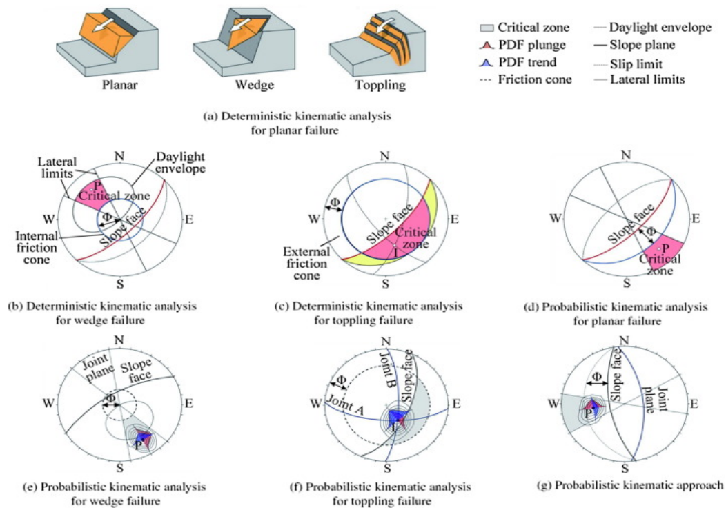
Figur 3: Strukturelle brotvilkår for planutgliding, kileutgliding og utvelting, dei rosa områda markerer instabilitet (Obregon og Mitri, 2019).
