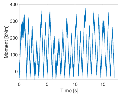
(d) Measurements of moment from Train 2.
