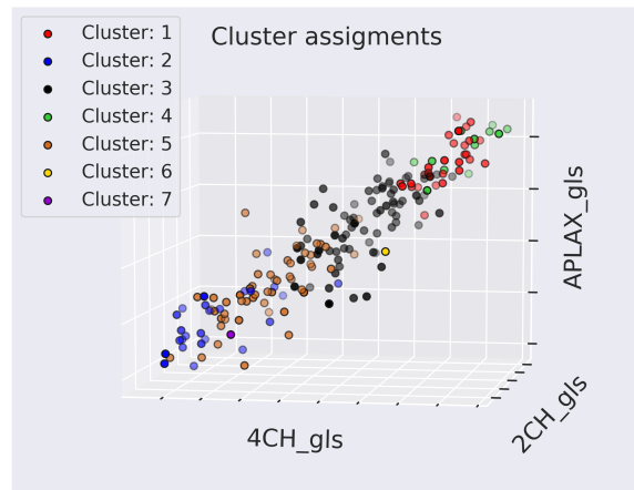
(d) GLS Average/7 cluster assignments.
