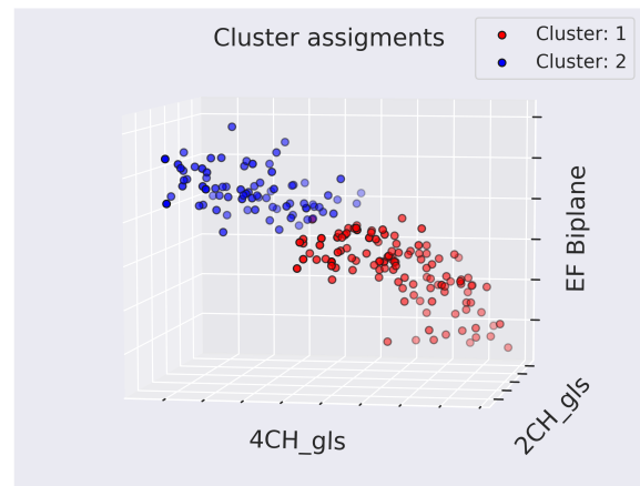
(d) Average/2 cluster assignments.
