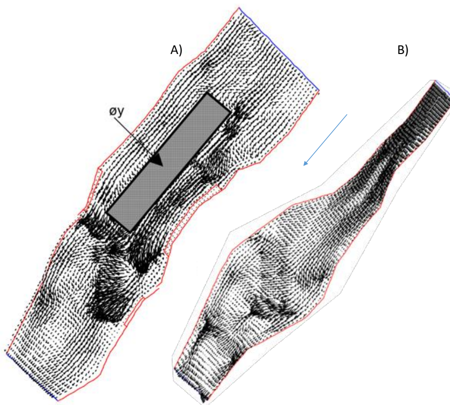
Fig. 35 Simulering av strømnig på strekninga på Nesheim med SSIIM, (A) viser tilhøve før tiltak og (B) visert situasjonen etter tiltak. Vassføringa er 1.3 \text{ m}^3/\text{s} . Øya som var i elva er blokkert ut ved simuleringa av situasjonen før tiltak (grått rektangel i A), medan denne delen av geometrien er heilt fjerna i tiltaksmodellen i B). Figurar frå Harby (2001). Pila viser straumretninga.
