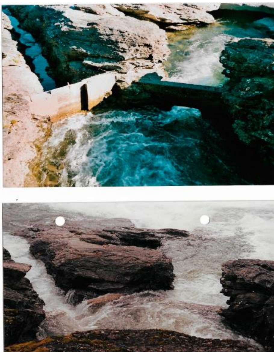
Fig. 58 Inngangene til trappa i Målselvfossen. På det nederste bildet vises det vanlige løpet til høyre og flominngangen til venstre. Det øverste bildet viser luka og inngangen fra Midtfallet i fossen, som benyttes når vannføringa i elva kommer under 60 \text{ m}^3/\text{s} og fisken kan gå et stykke opp i fossen. Foto: Helge Utby.
