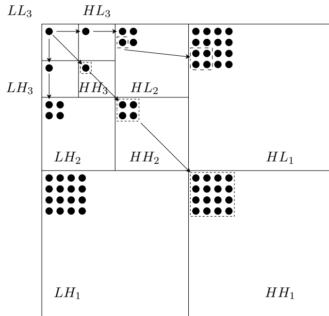
Figur 2.8: “Zerotree” koding på bilde dekomponert med oktavbånd filterbank. Figuren viser avhengigheten mellom forelderpixel og barnpixel, hvor hvert forelderpixel på ett nivå har fire barnpixel i det neste nivået i trestrukturen.
