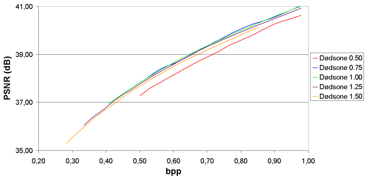
Figur 5.5: Figuren viser hvordan dødsone størrelsen påvirker bpp - PSNR kurven for sekvensen foreman . Bufferstørrelsen er satt til 8 rammer.
