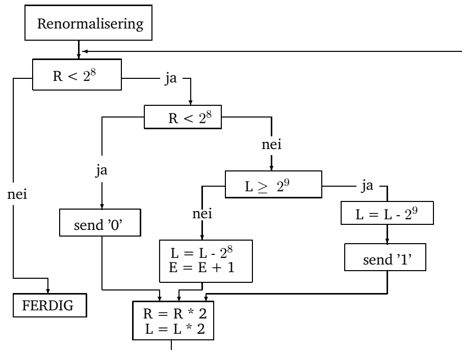
Figur 3.7: Renormalisering i CABAC-koder. L =nedre grense på intervallet, R =bredden på intervallet og E =etterfølger bit som beskrevet i 2.9. Figuren er laget etter en skisse i [14]
