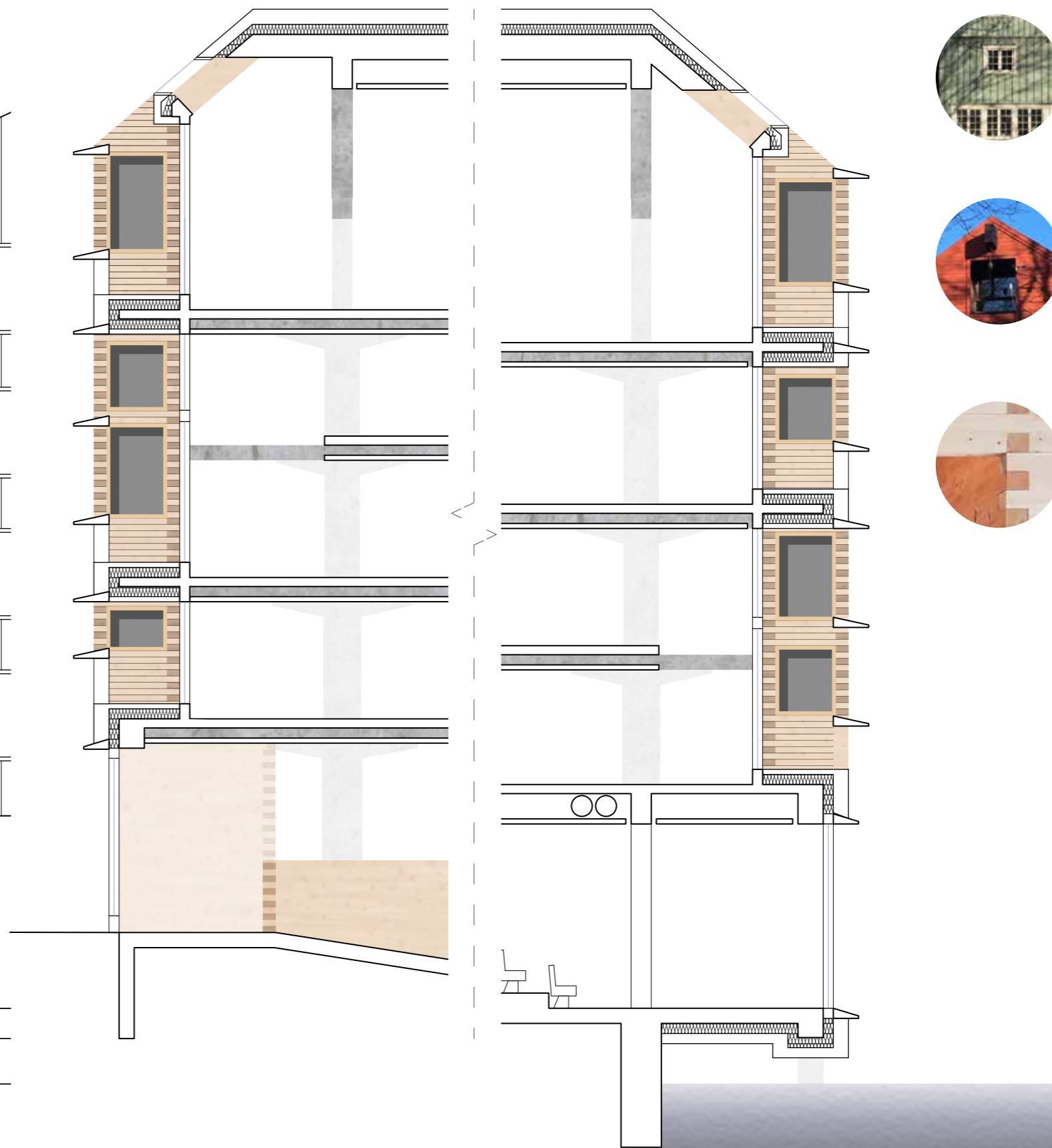
Fasadesnitt Bar og Scene brygge
