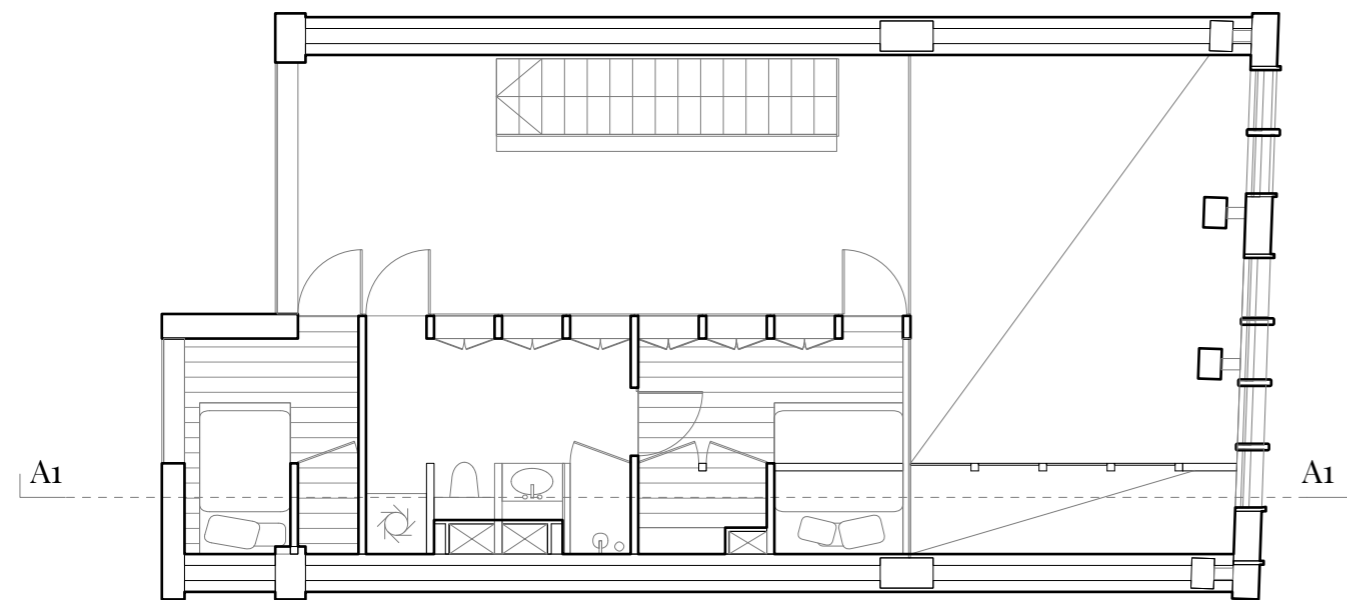
Plan 4, Leilighetstype 1, dobbelthøy
