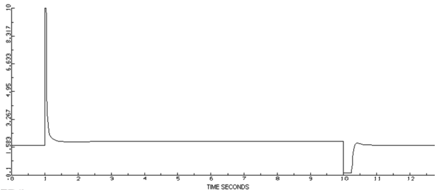
Figur 18: Tidsrespons for VR, feltspenning i feltgenerator ved redusert KI
