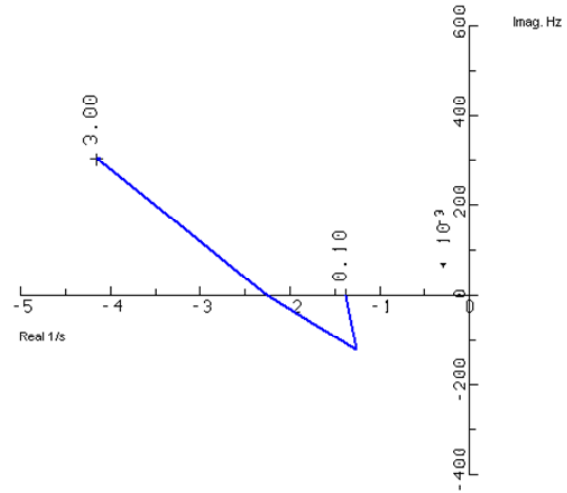
Figur 39: Data scanning av egenverdiparet 22/23 når KA i EXC DG1 varieres mellom 0.1 og 3p.u
