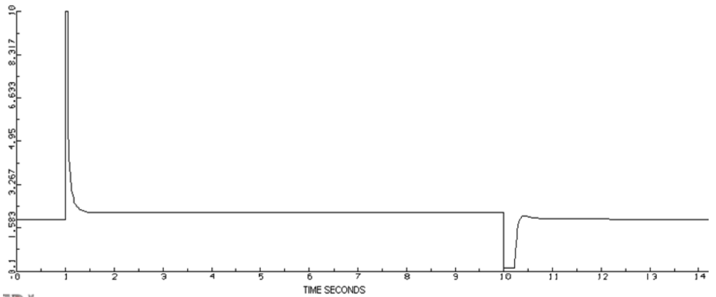
Figur 6: Tidsrespons for VR, feltspenning i feltgenerator ved økt KP
