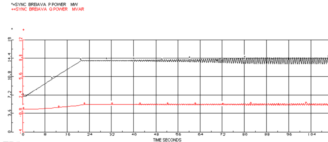
Figur 59: P og Q til synkrogenerator Breiava med spenningsregulator nr.1 (KA=1p.u) med H=2 ved økning i turbinmoment fra 7 MW til 14MW
