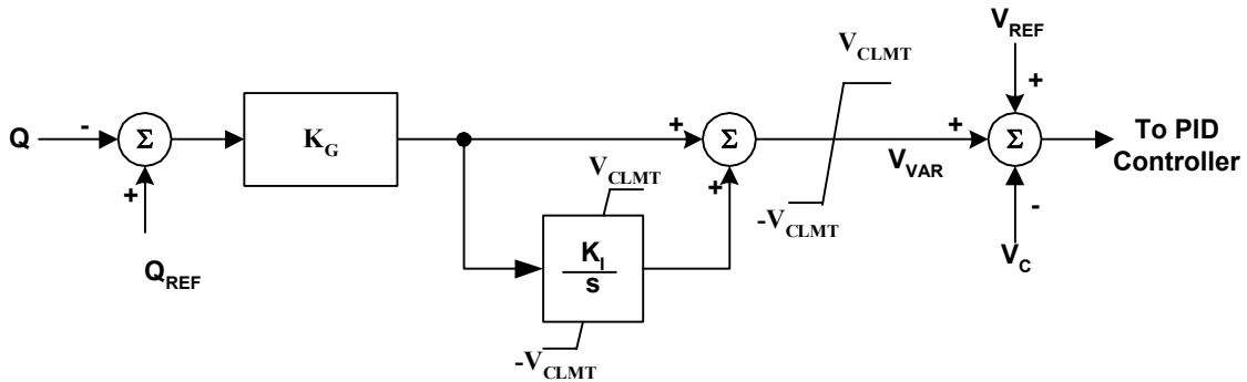
Figur 15: Blokkdiagram for VAR kontroll type 2 [21]
