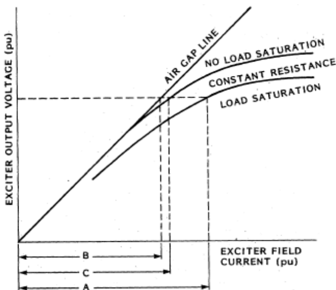
Figur 18: Metningskarakteristikk for feltgenerator [27]
