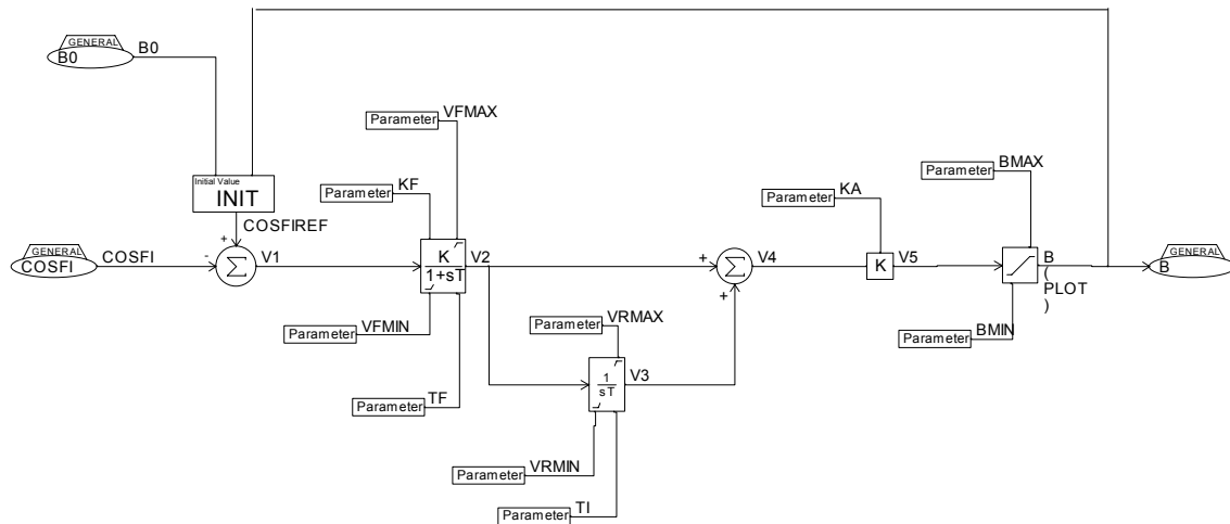
Figur 2: Blokkdiagram for CREG.
