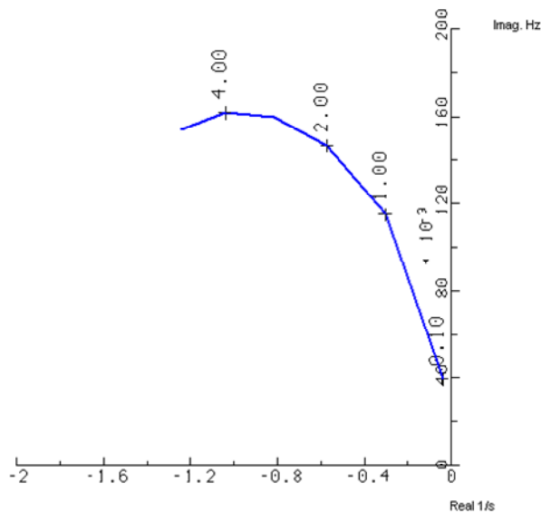
Figur 40: Data scanning ved endring av KA fra 0.1 til 5 p.u for egenverdi 26
