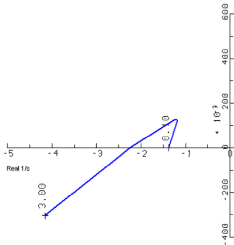
Figur 39: Data scanning av egenverdiparet 22/23 når KA i EXC DG1 varieres mellom 0.1 og 3p.u
