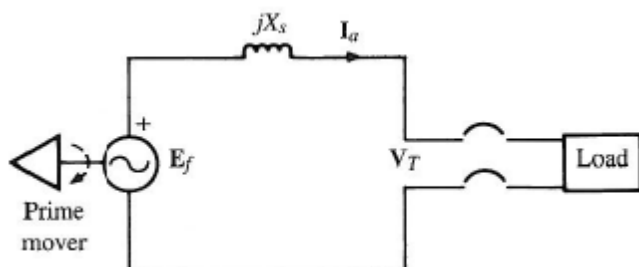
Figur 8: Enlinjeskjema og for en synkrogenerator med sylindrisk rotor [12]
