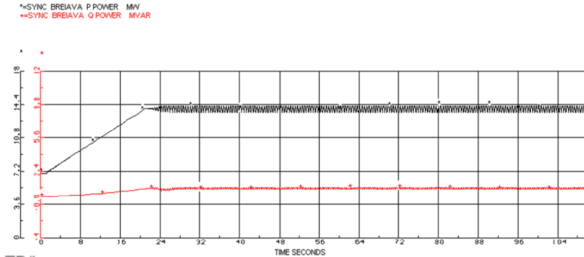
Figur 58: P og Q til synkrogenerator Breiava med spenningsregulator nr.1 med KA=3 ved økning i turbinmoment fra 7 MW til 14MW
