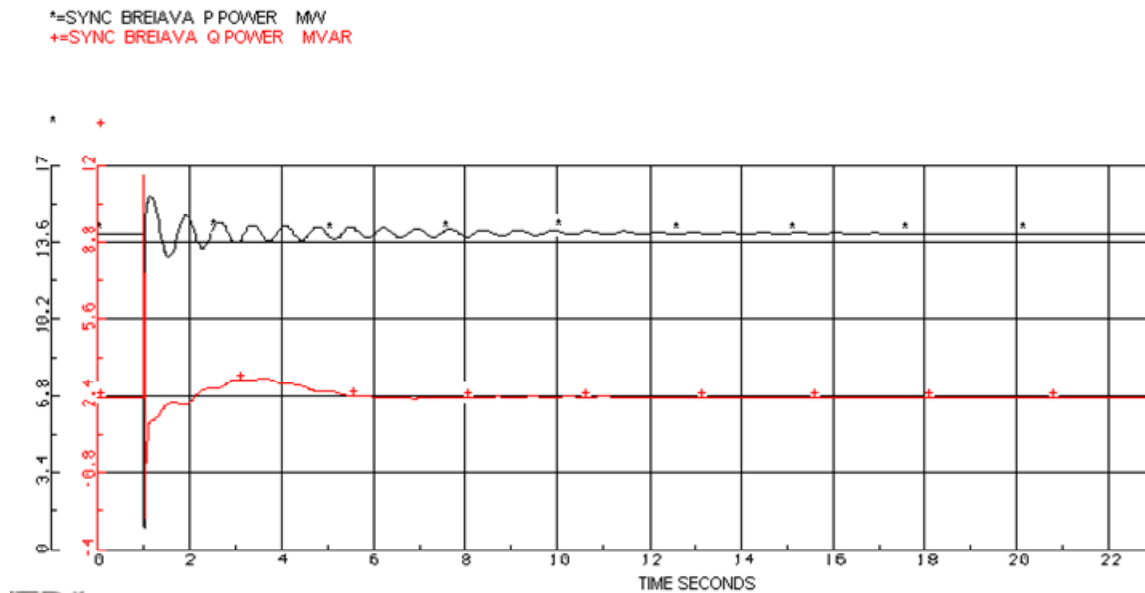
Figur 56: P og Q til synkrongenerator Breiava med spenningsregulator nr 1 KA=1p.u og H=2s ved feil på node LYSES22.
