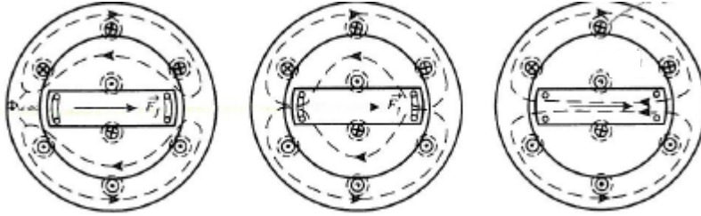
Figur 10: Veien til statorfluksen i en synkrogenerator ved sub transient (t.h), transient og stasjonær tilstand
