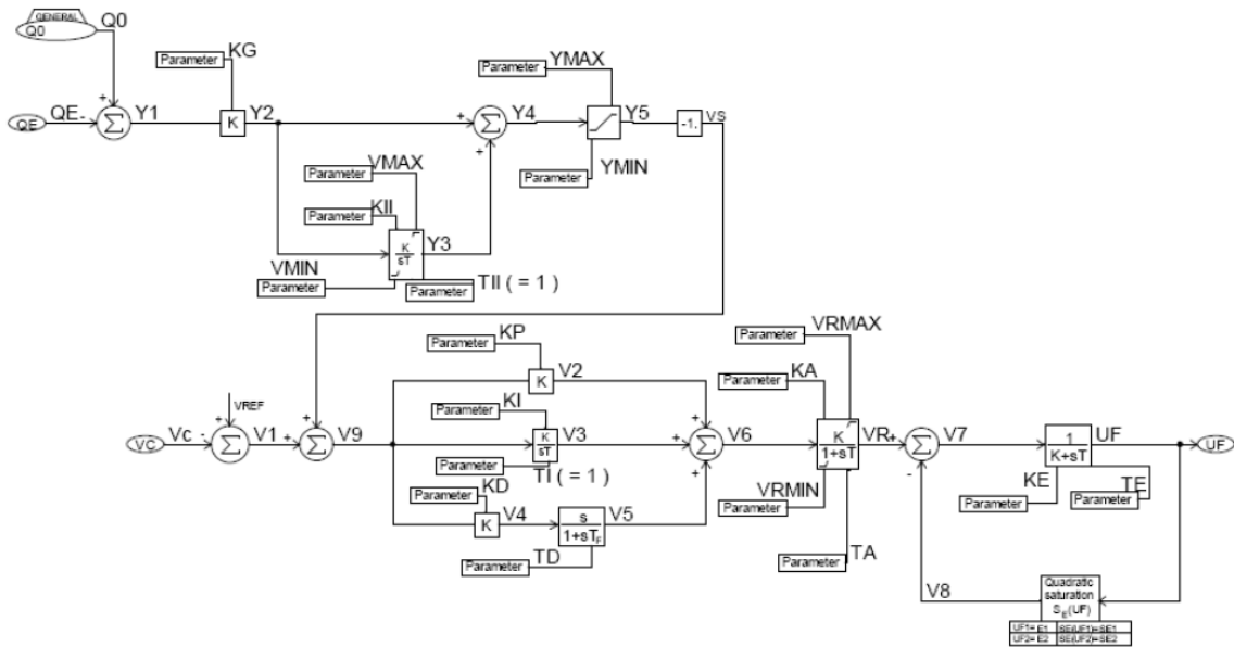
Figur 21: Blokkdiagram av EXCITERQE tegnet i HiDraw
