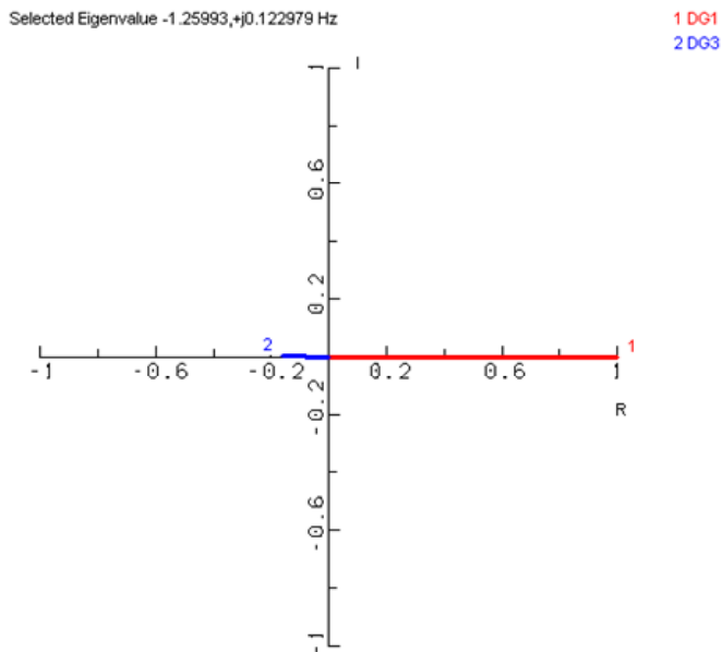
Figur 36: Modal analyse av egenverdi 22: -1,2599+j0,1298
