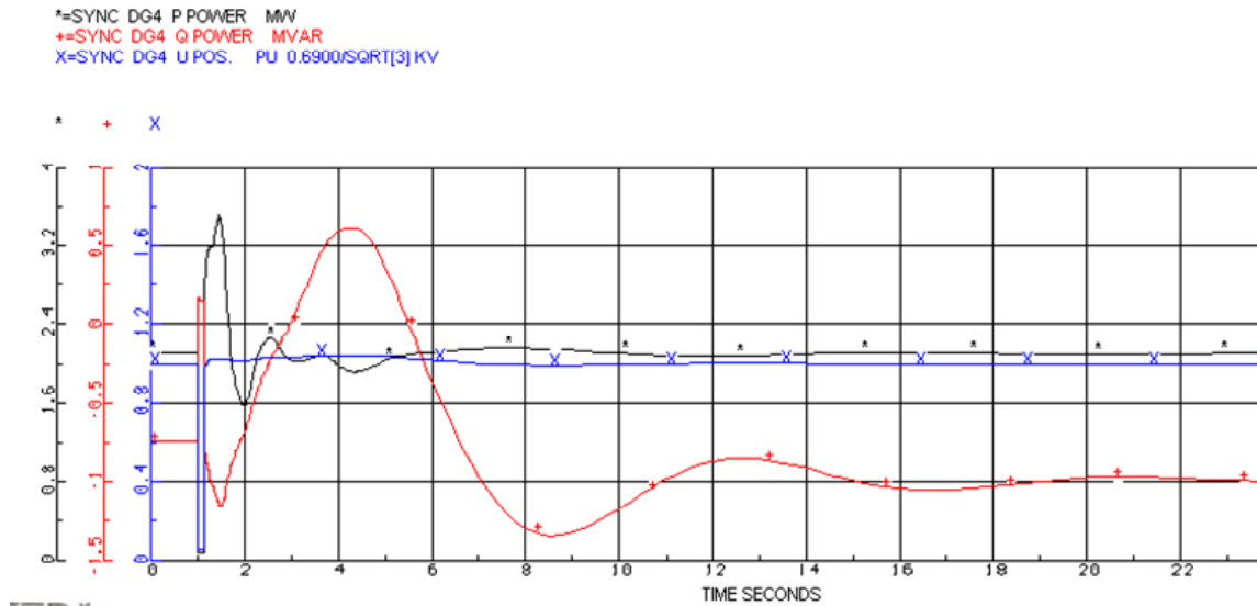
Figur 45: P, Q og U til DG4, med H=2, ved kortslutning på node BUS9.
