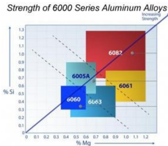
Fig.24 Aluminium Alloys 6xxx serie
