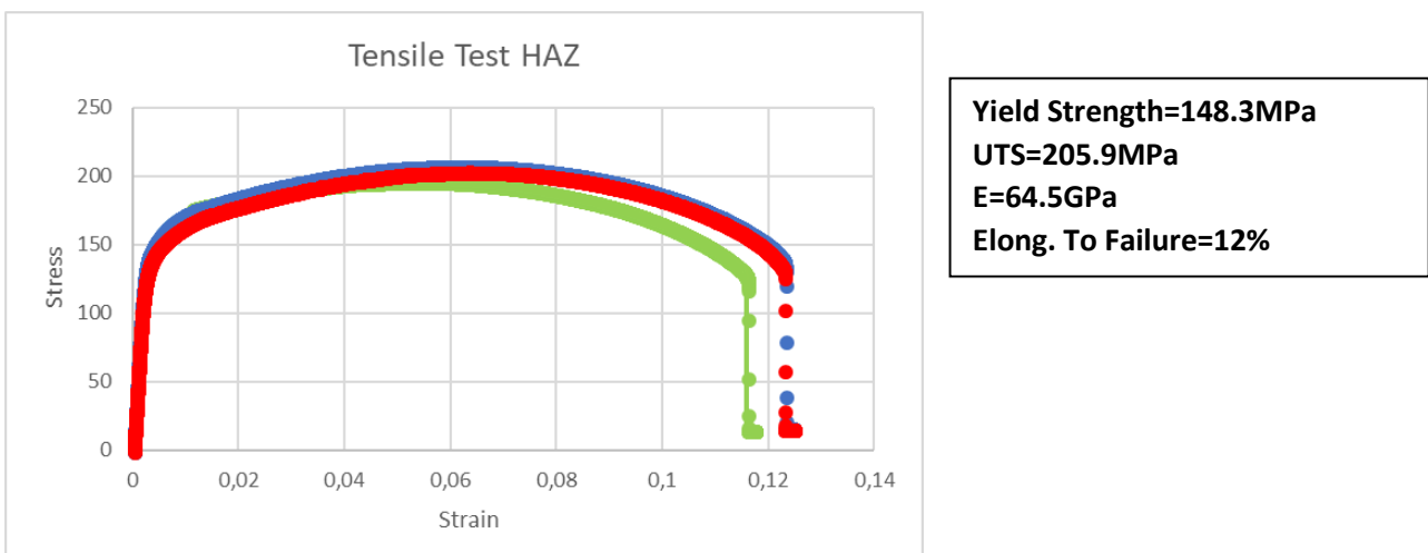
Fig.70 tensile test HAZ
