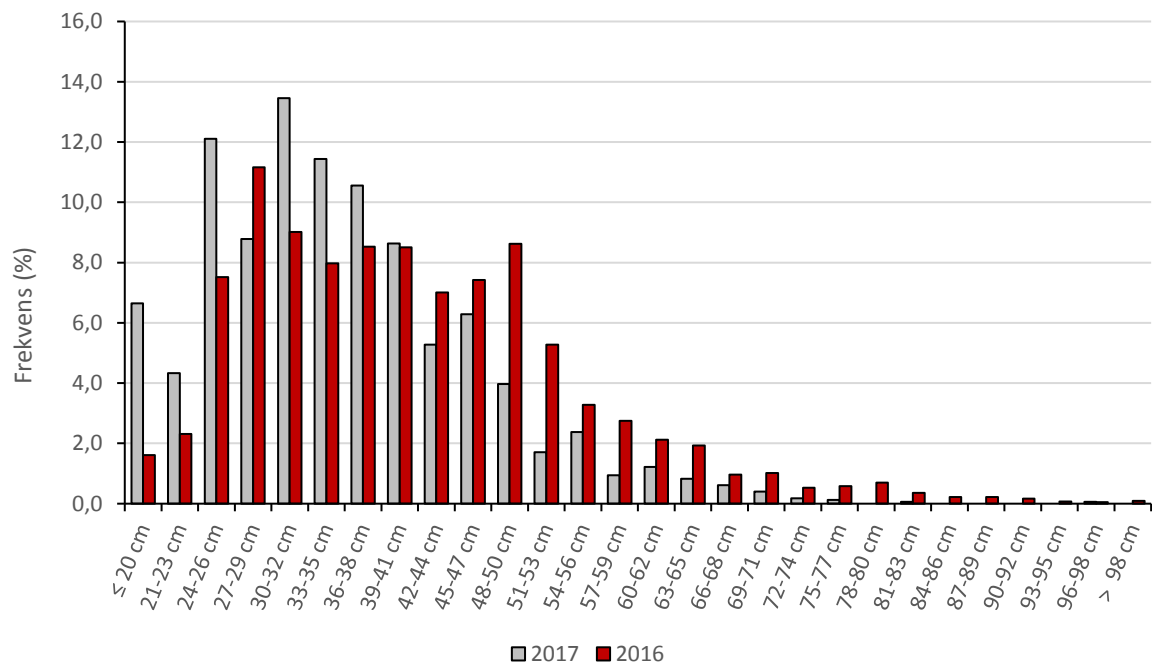
Figur 22. Størrelsesfordelingen (kroppslengde i cm) for sjørørret som vandret opp i 2016 sammenlignet med størrelsesfordelingen registrert oppvandrende sjørørret i 2017 registrert i videoovervåkingen på Ureidet i Ur-voldvassdraget.
