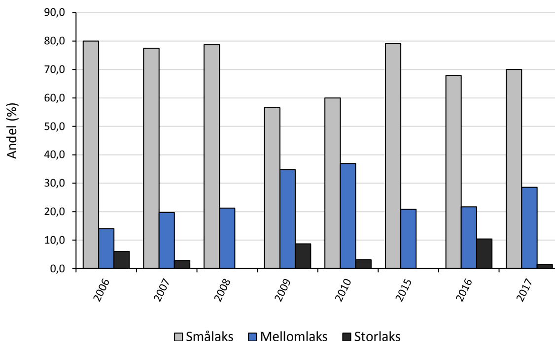
Figur 20. Fordeling av små-, mellom- og storlags registrert i videoovervåkningen på Ureidet i Ursvoldvassdraget i årene 2006-2010 og 2015-2017.
