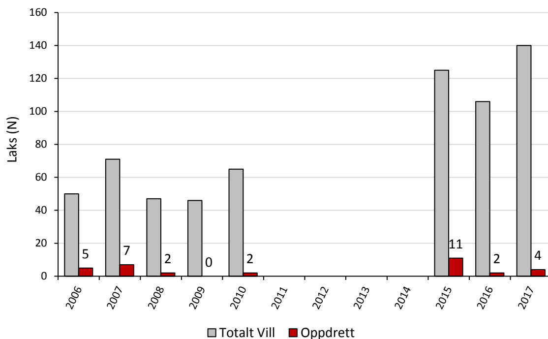
Figur 19. Antall netto oppvandrende vill- og oppdrettslaks registrert i videoovervåkningen på Ureidet i Ursvoldvassdraget i årene 2006-2010 og 2015-2017.
