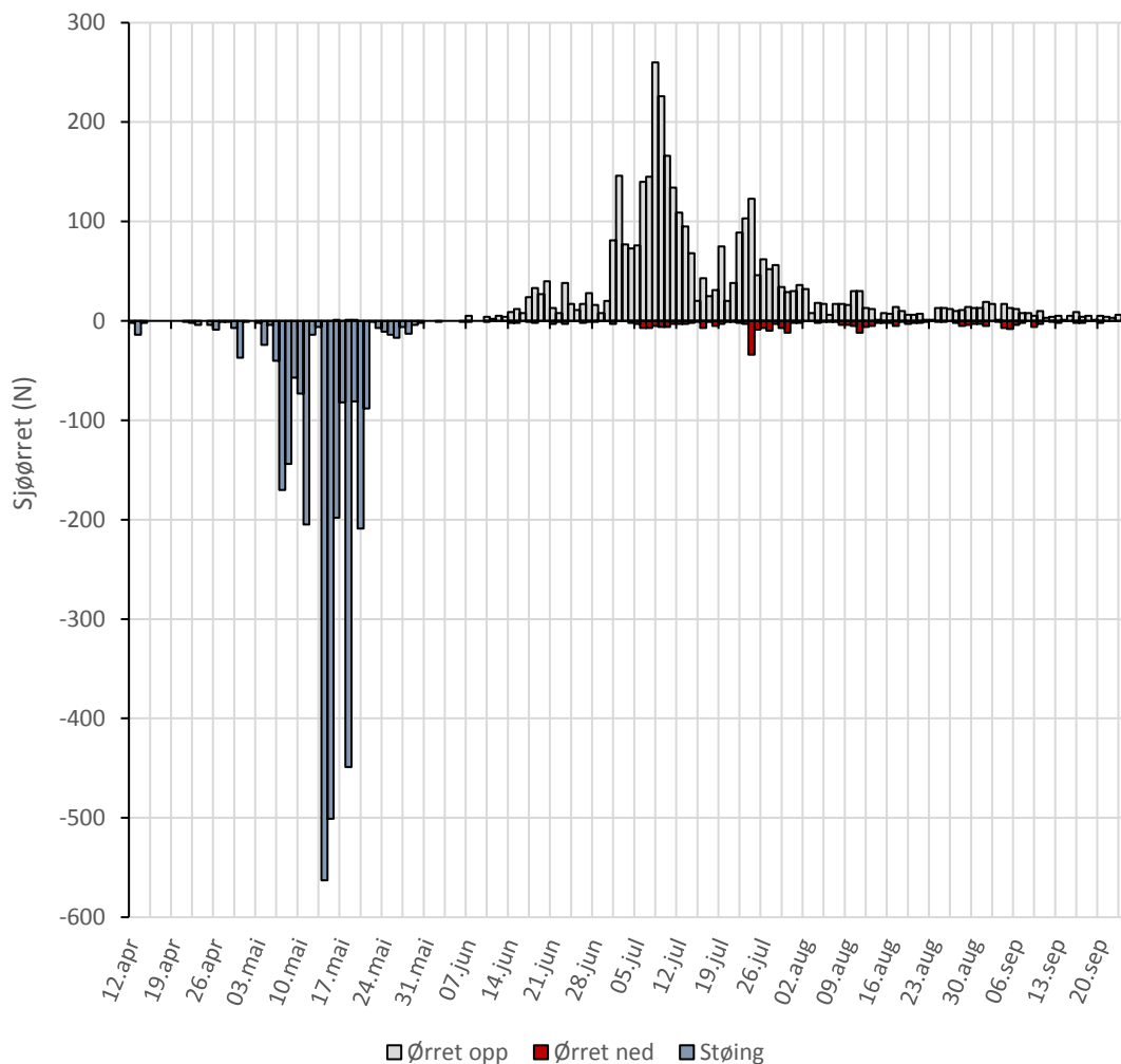
Figur 24. Utvandring av støing av sjørret og oppvandring av sjørret fra sjøen registrert i videoovervåkingen på Ureidet i Ursvoldvassdraget i 2017.
