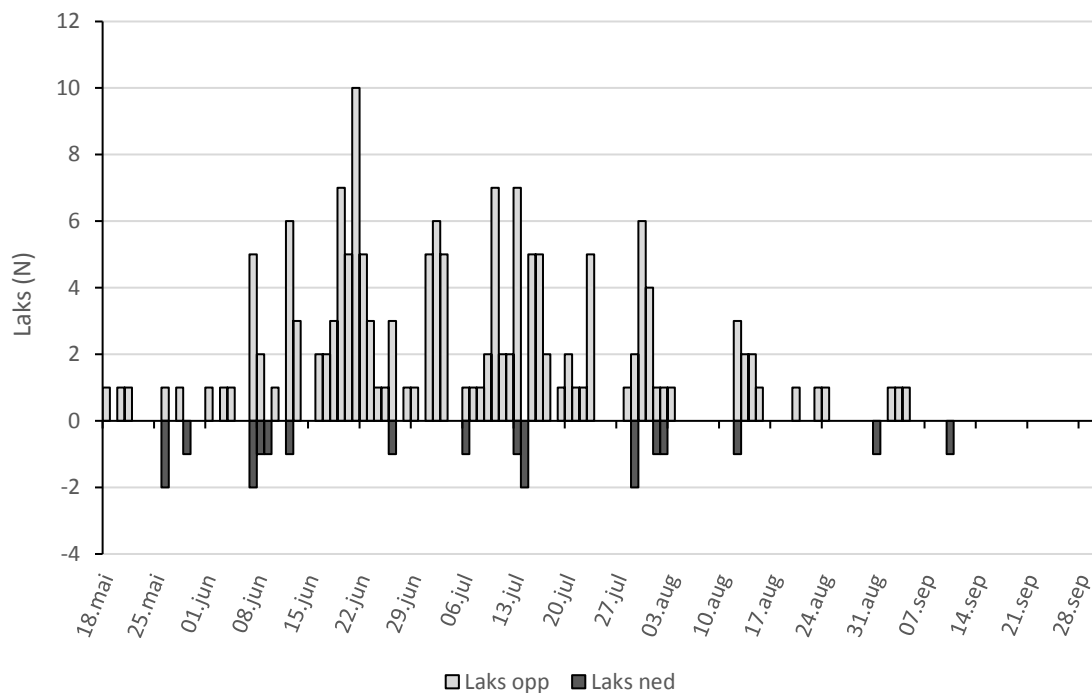
Figur 18. Antall opp- og antatt midlertidig nedvandrende laks registrert i videoovervåkningen på Ureidet i Ursvoldvassdraget i 2017.
