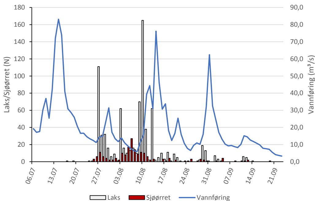
Figur 7. Antall oppvandrende laks (hvit) og sjøørret (rød) per dag registrert på video i Brattfossen (Åbjøravassdraget) 2017. Vannføringen målt ved NVE sin målestasjon ved utløpet av Åbjørvatnet er angitt med blått.
