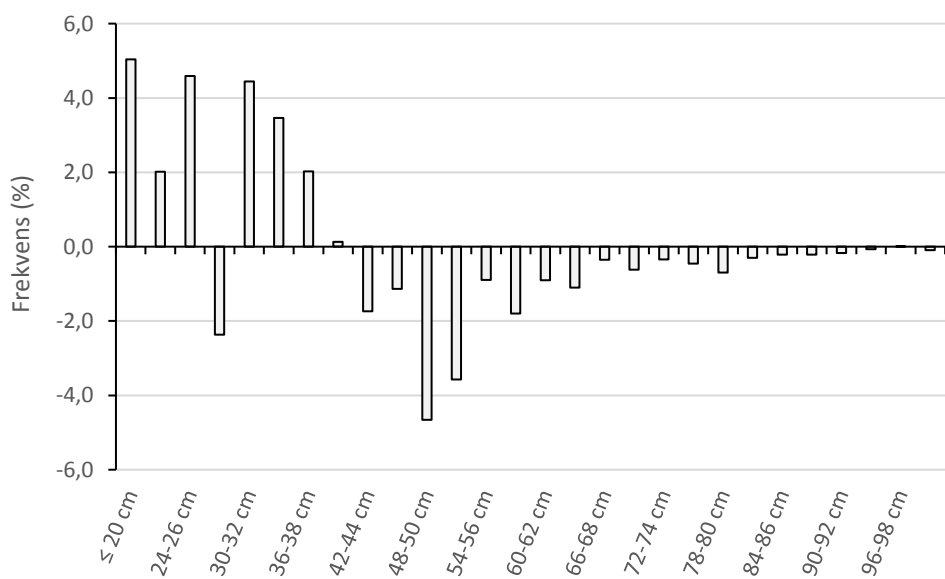
Figur 23. Differansen i størrelsesfordeling (frekvens i 2017 minus frekvens i 2016) mellom oppvandrende sjørørret i 2017 og 2017, registrert i videoovervåkingen på Ureidet i Ur-voldvassdraget.
