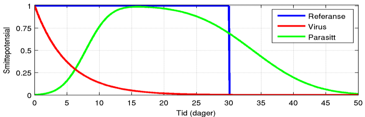
Figur 31. Framstilling av smittepotensial-kurven for bruk for levetidsberegning for patogener.
