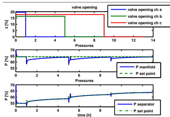
Fig. 8. Welltest results
