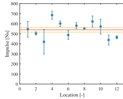
(d) Impulse I
