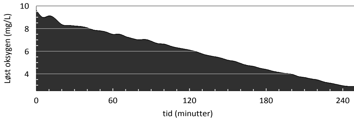
Figur 2.4: Fall i løst oksygen ( \text{mg O}_2 \text{ L}^{-1} ) ved bergnebb's samlede forbruk i lukket måleoppsett 4 timer. Måling utført januar med 33 liter sjøvannvann. Vekt: 32,7 \text{ g. } (\pm 14,7) . n=18 .
