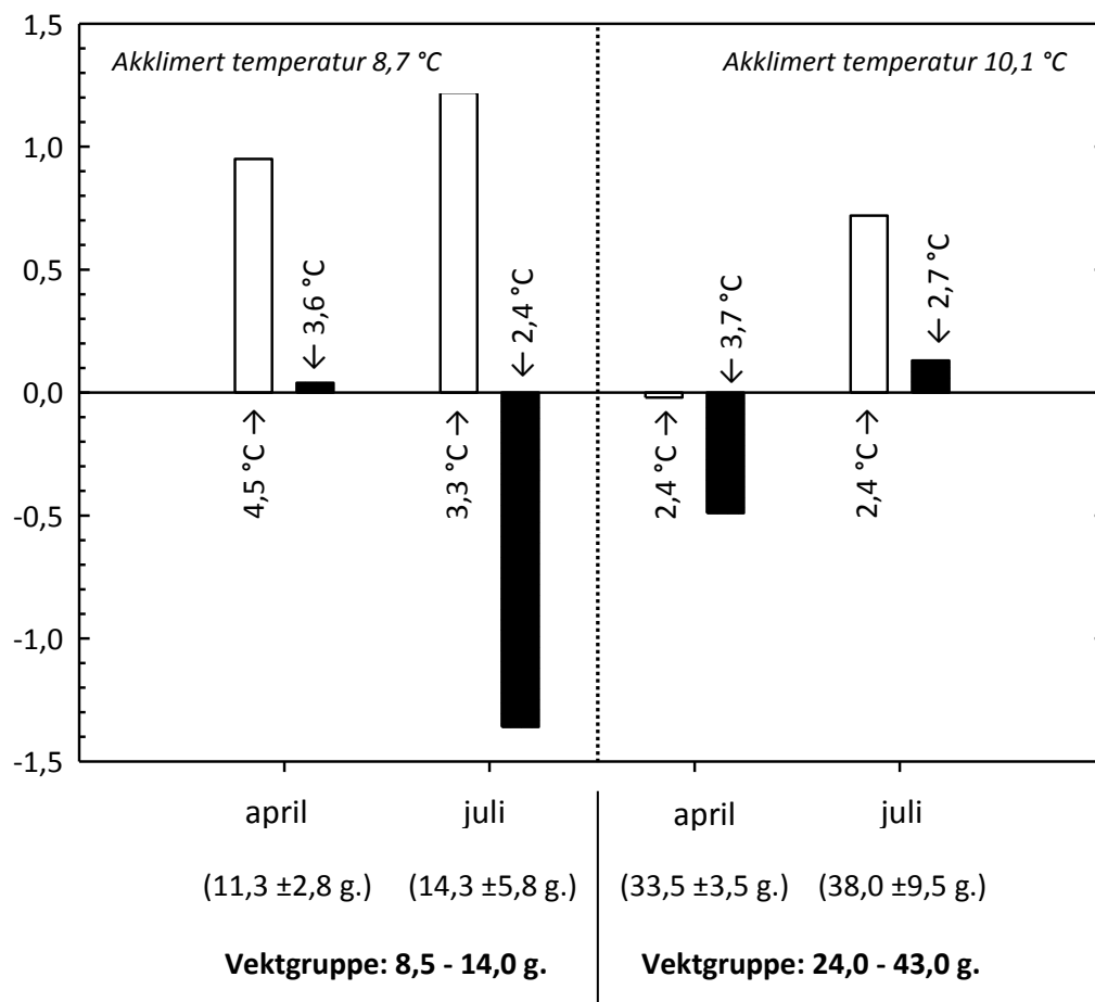
Figur 3.5: Oksygenforbruk for vektgrupper av små og store bergnebb målt i april og juli. Søyler viser differanse i oksygenforbruk ved akutt økning/senkning i temperatur til forskjell fra oksygenforbruk hos samme gruppe ved akklimert oppholdstemperatur. n=10 for alle forsøksgrupper.
