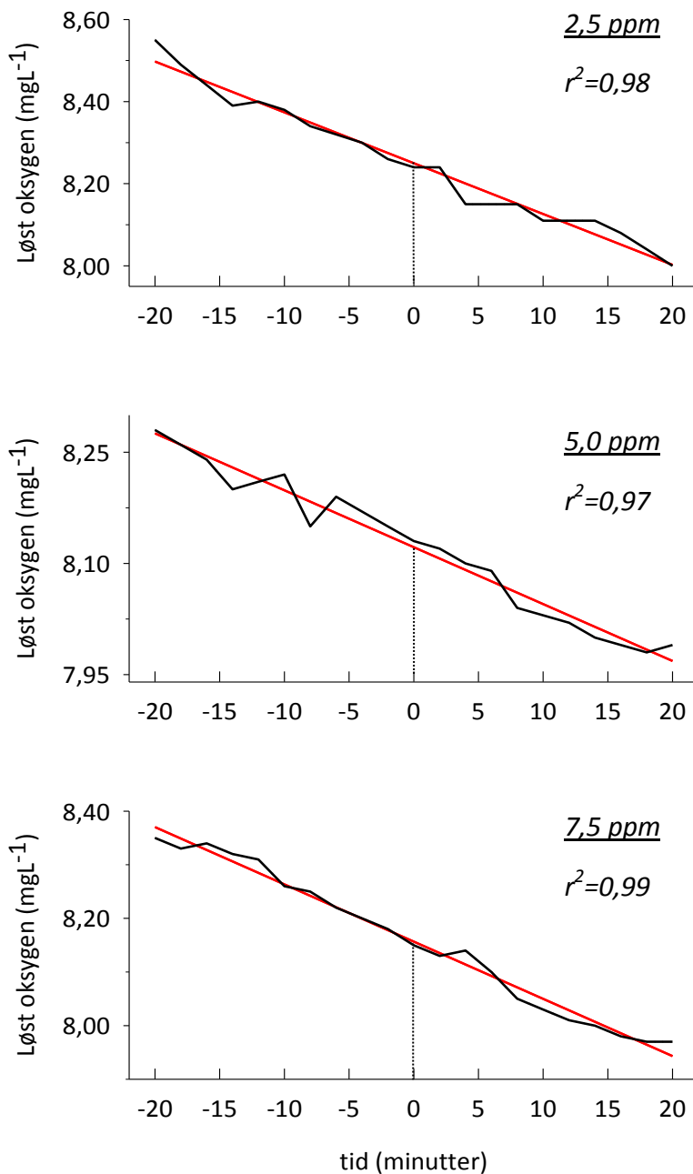
Figur 3.9: Fall i løst mengde oksygen ved grupper av bergnebb opphold i forsøksenhet. Fra tid 0 (stiplet linje) er tilført Aqui-S; 2,5- (75 \mu\text{l} ), 5,0- (150 \mu\text{l} ) og 7,5 ppm (225 \mu\text{l} ). Lineær regresjonslinje (rød) vist for hele oksygenkurven, med 99 % konfidensintervall og regresjonskoeffisient ( r^2 ). n=10 for hver gruppe.
