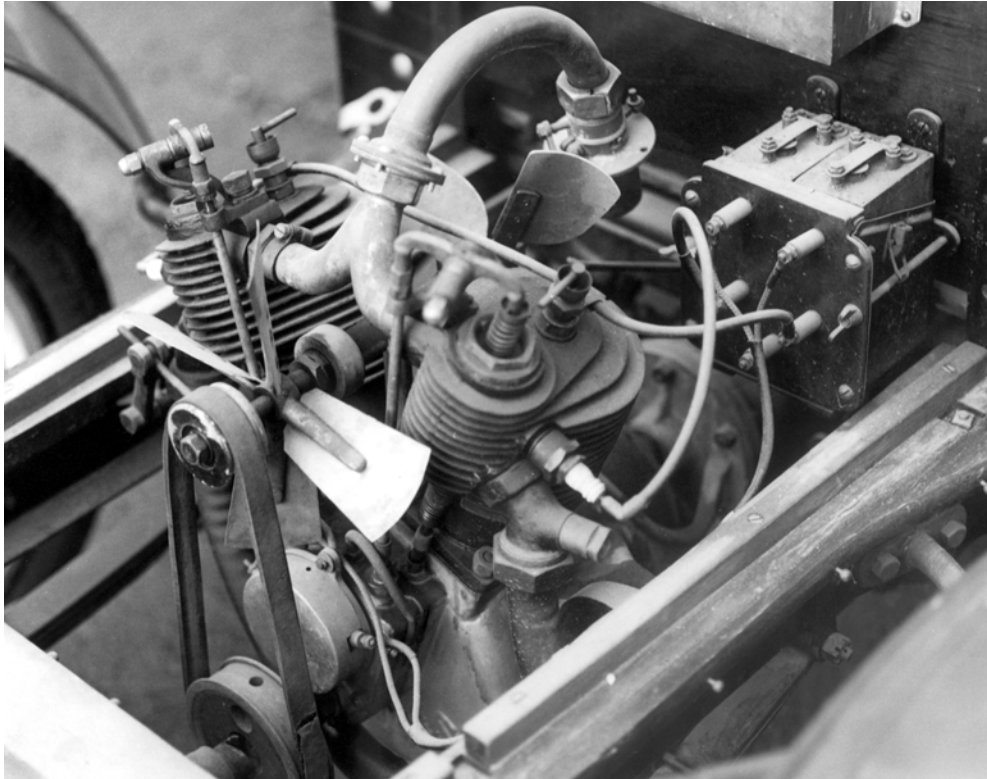
Piccoloens motor, en luftavkjølt bensindrevet V-2 som like gjerne kunne ha stått i en motorsykkel fra den samme perioden. Dette forteller om uklare teknologiske skillelinjer. Samtidig peker teknologivalget i retning av at lav vekt var viktigere enn fart.
