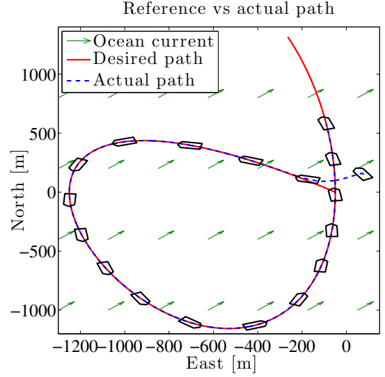
Fig. 4: Desired and actual path C_2 .
