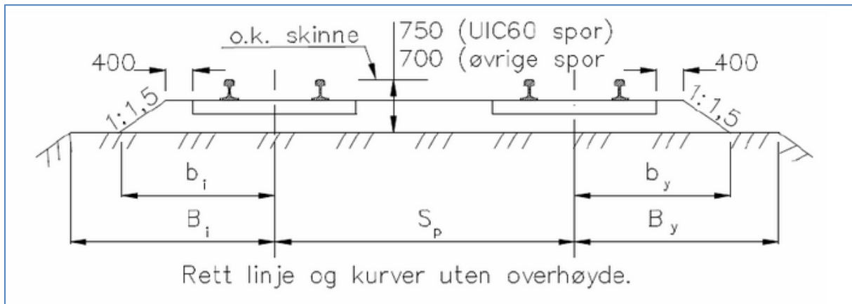
Figur 23 – Standard ballastprofil som skal anvendes for dobbeltspor 45
