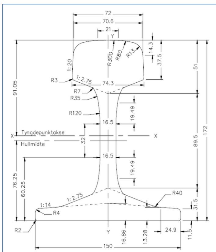
Figur 20 – Skinneprofil 60E1 42
