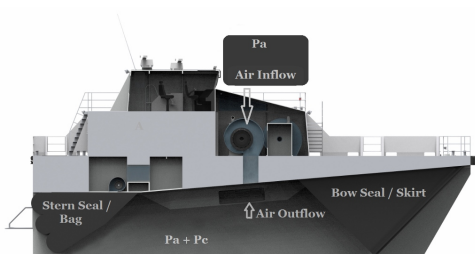
Fig. 1. The SES Concept (Umoe Mandal (UM) Proprietary)
