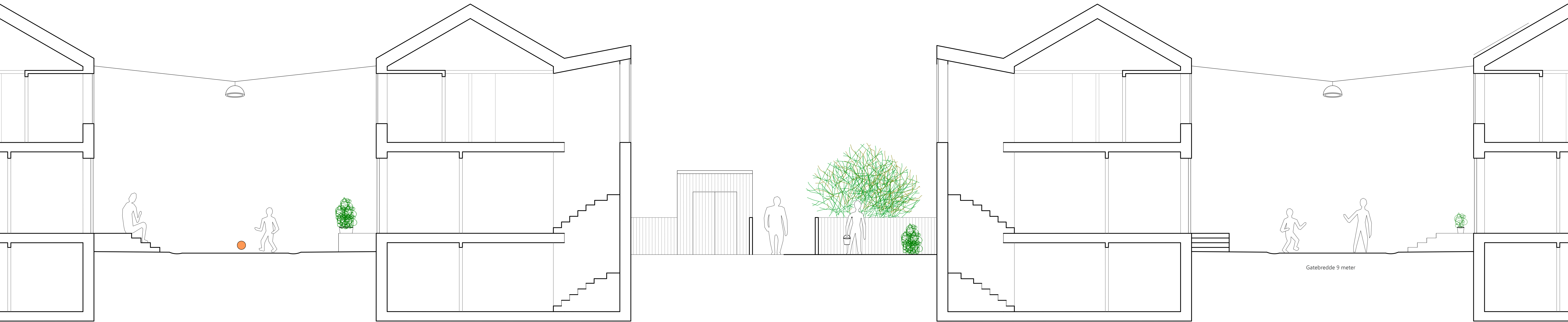
Typisk snitt gjennom gate og bakgård, 1:50.
