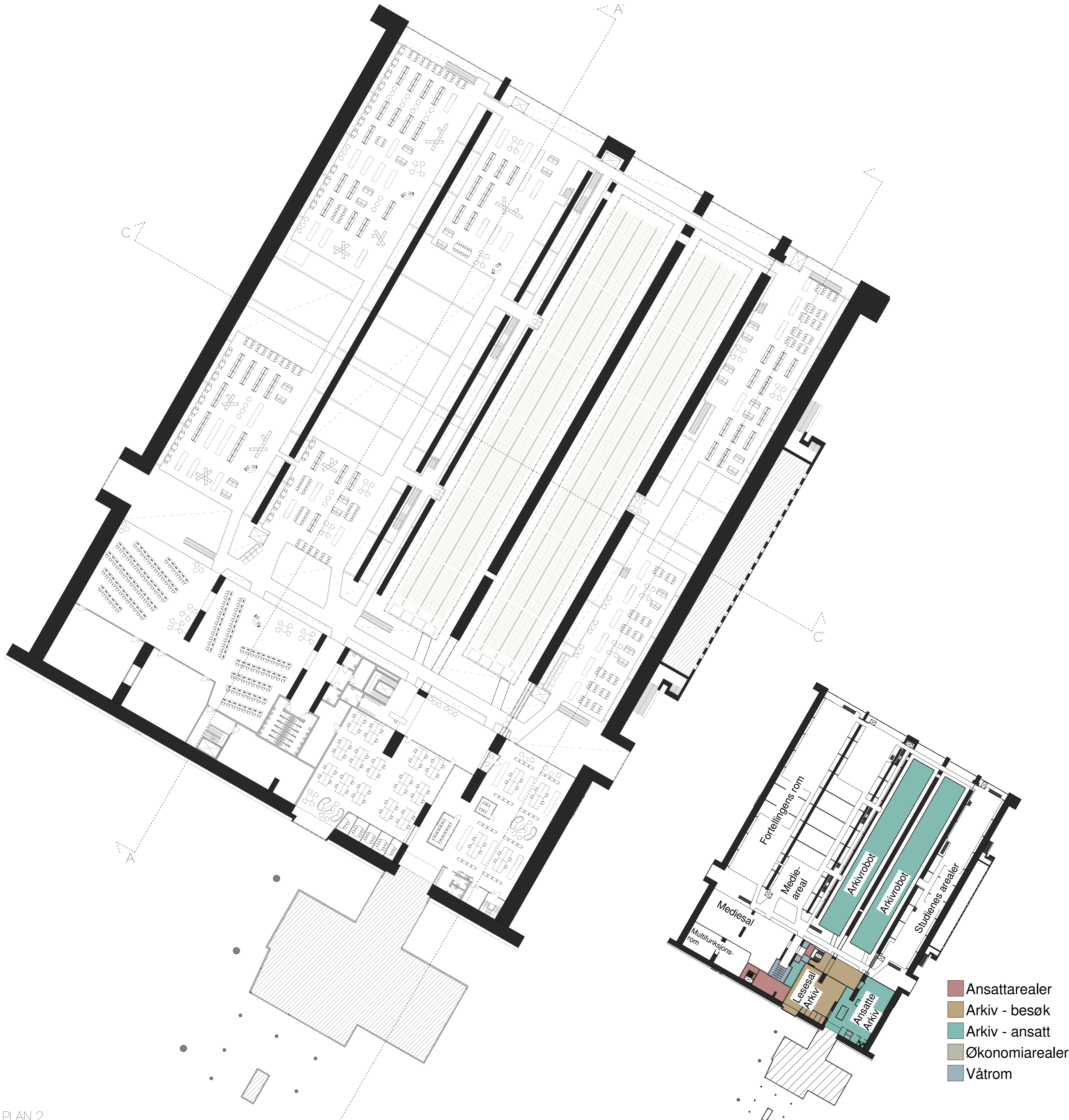
PLAN 2 M 1:100
