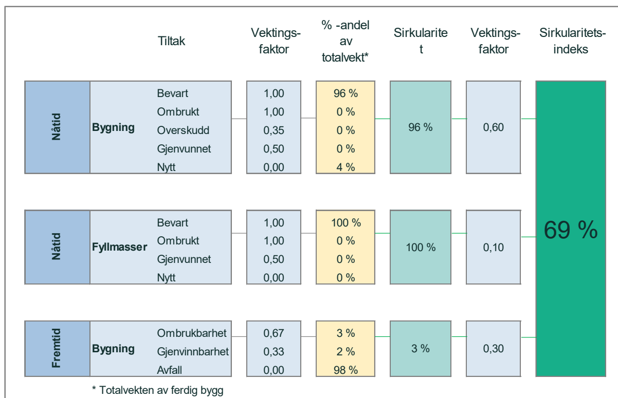
Figur 14. Resultat fra FutureBuilds sirkularitetsindeks for ett av boligprosjektene: Kristian Augusts gate 23 (KA23).
