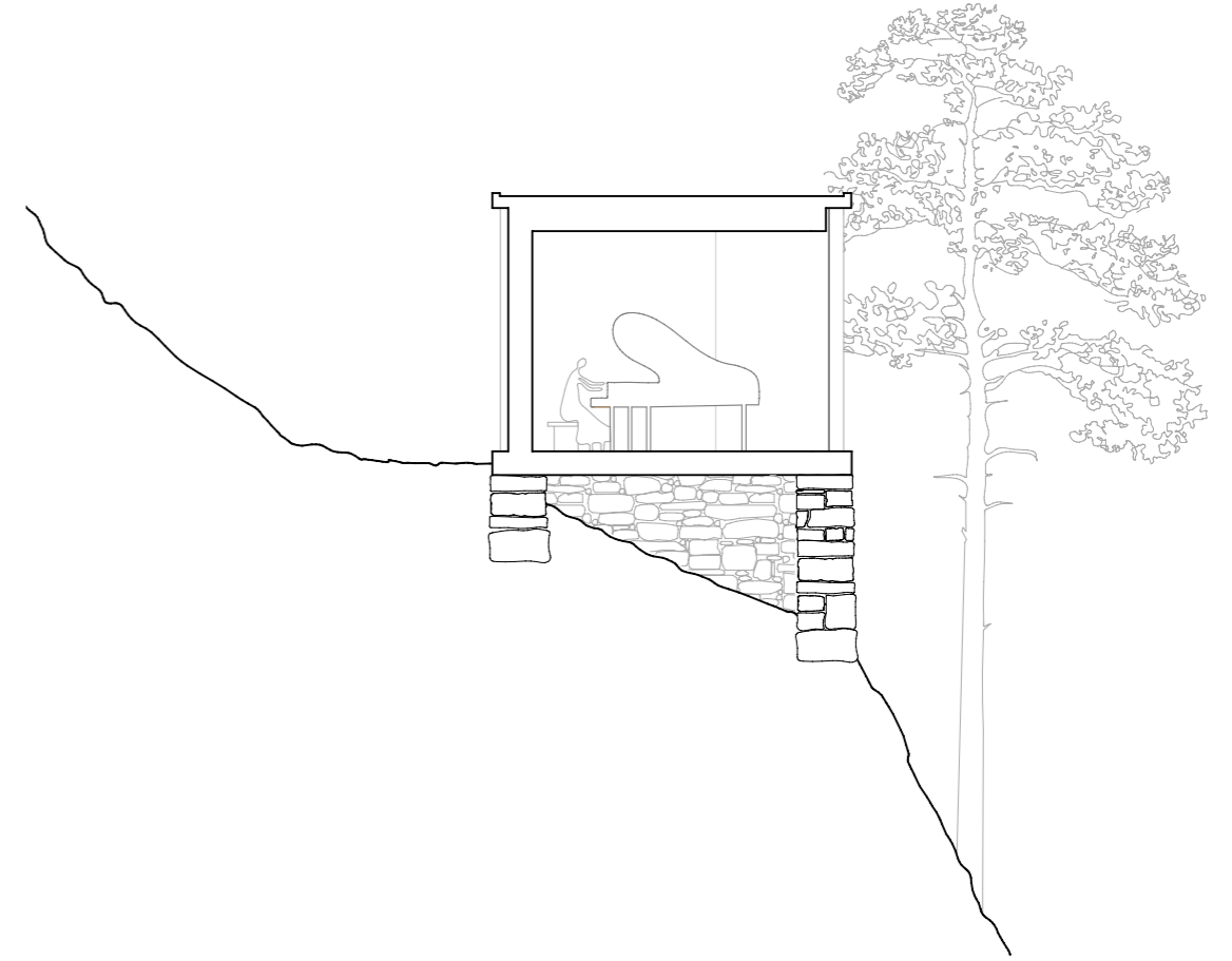
Snitt nn'
