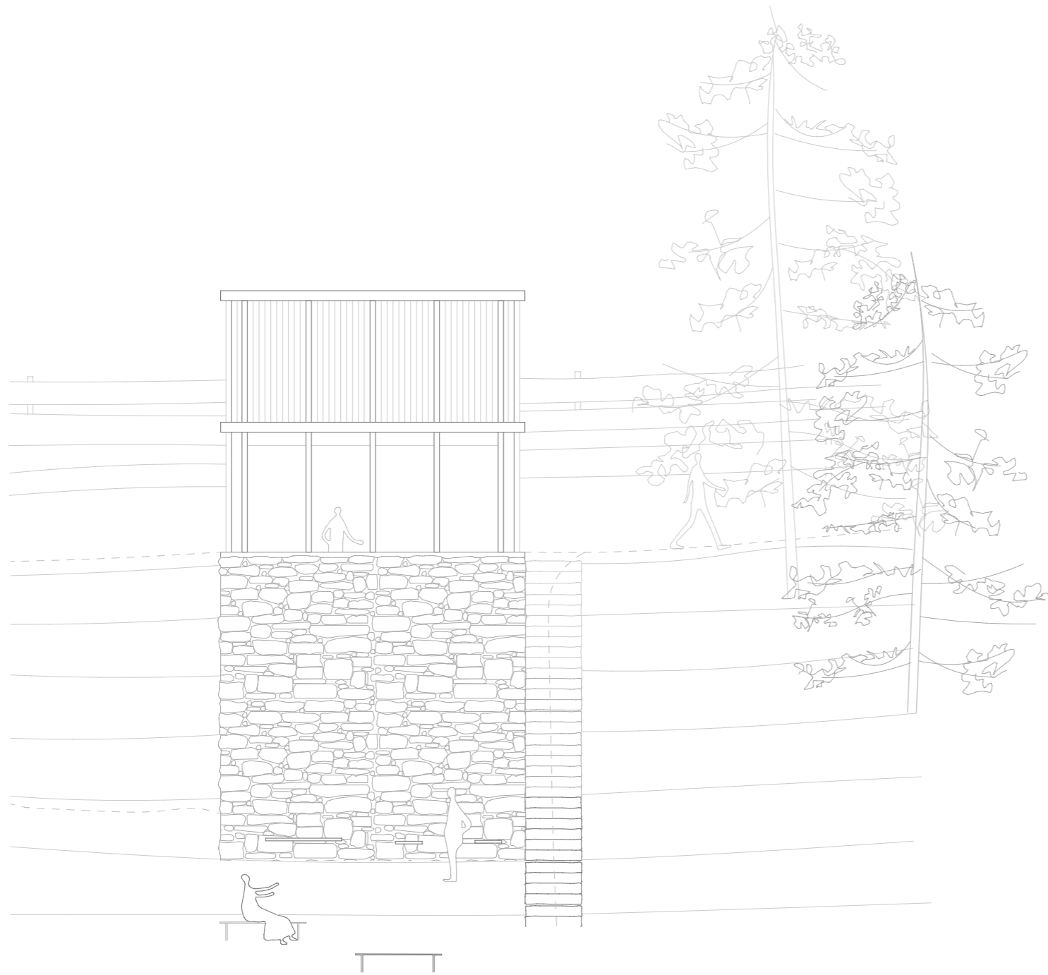
Fasade sør
