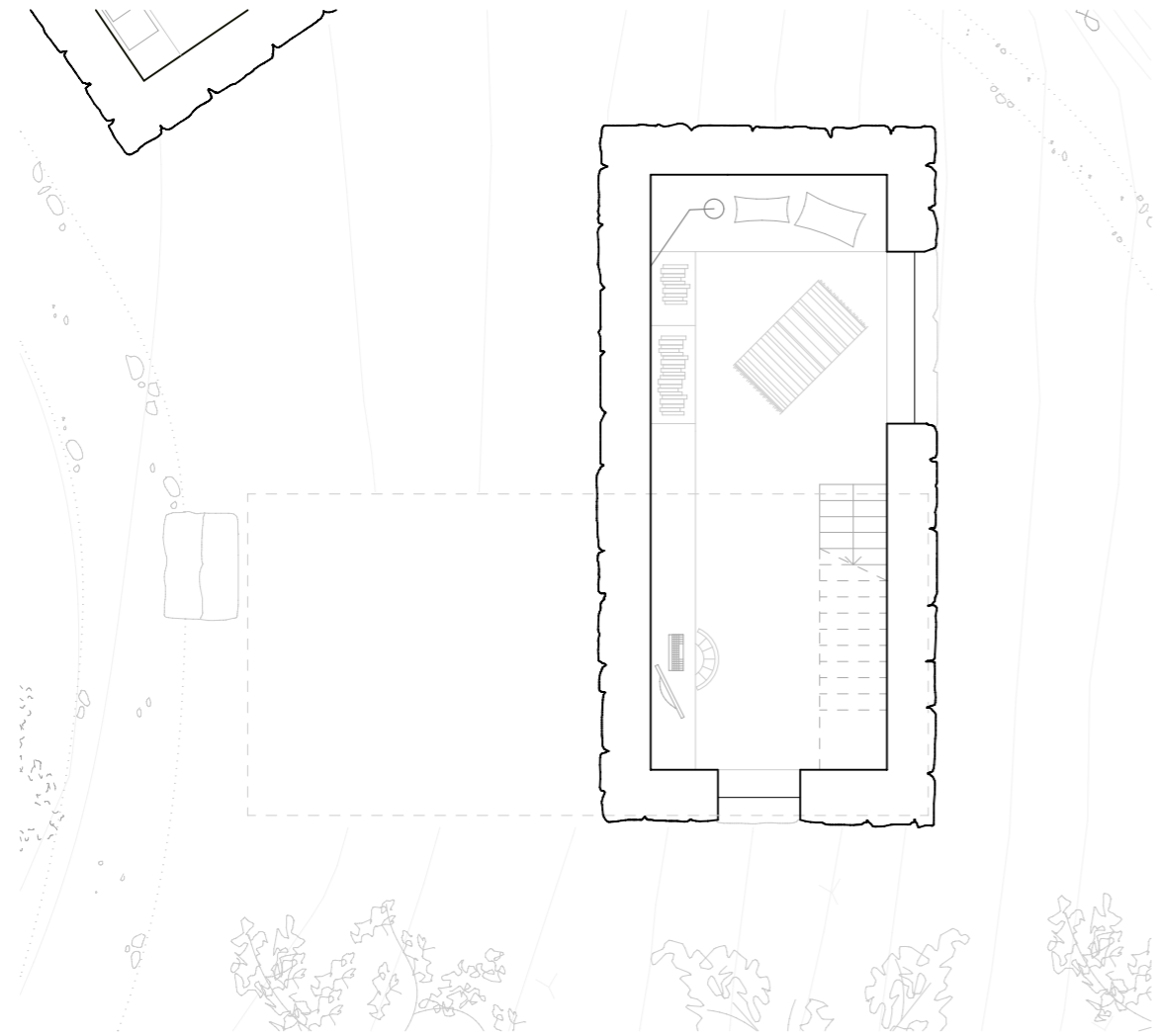
Plan 1. etg
