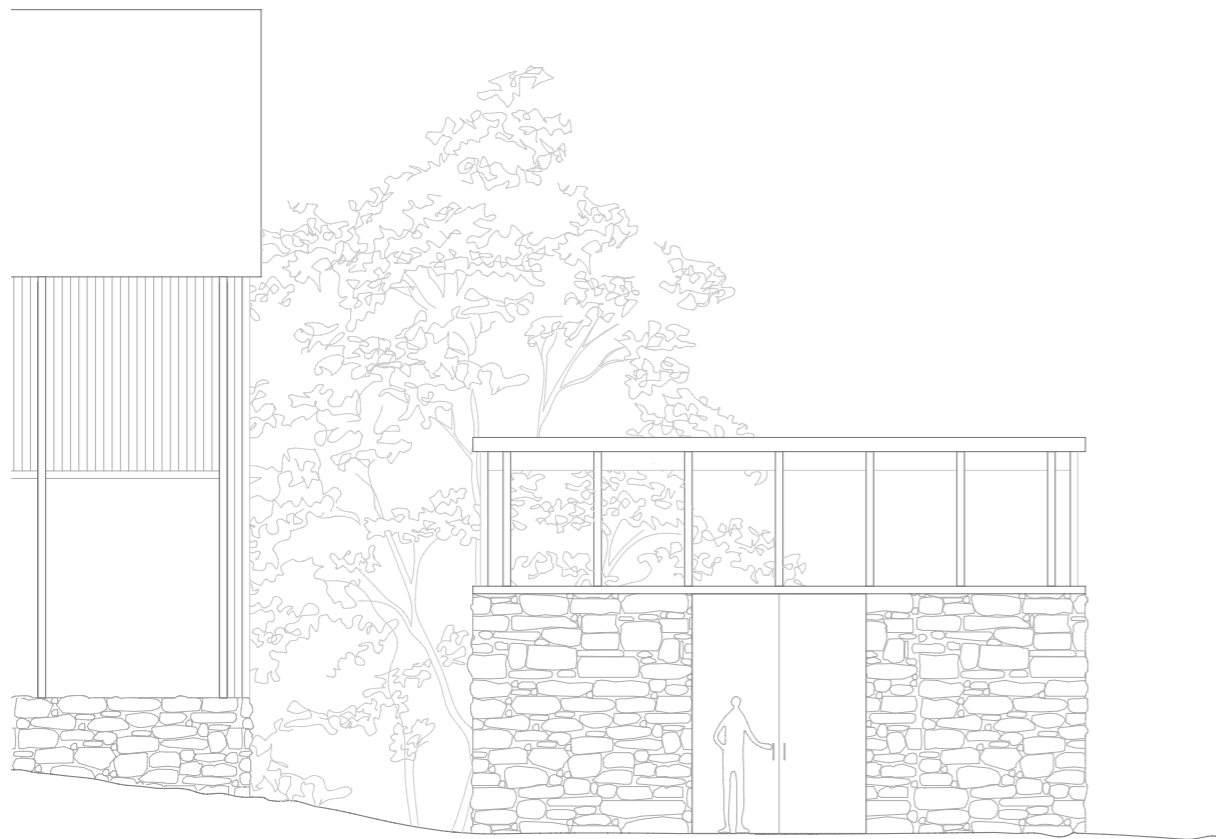
Fasade vest
