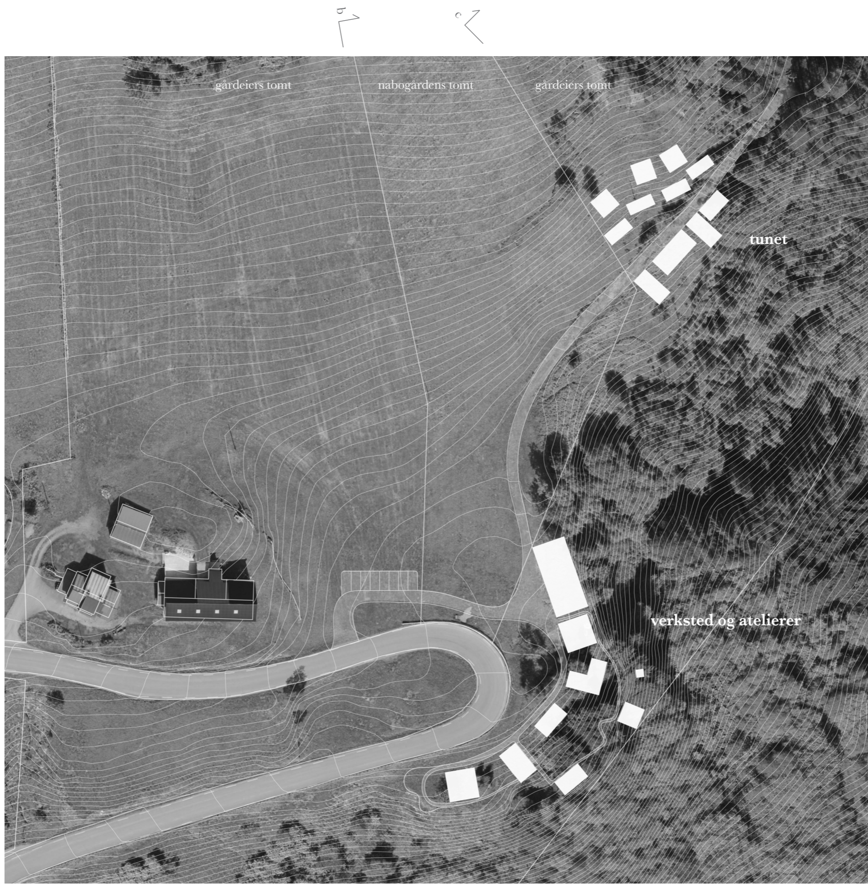
Situasjonsplan 1-1000 ☺
