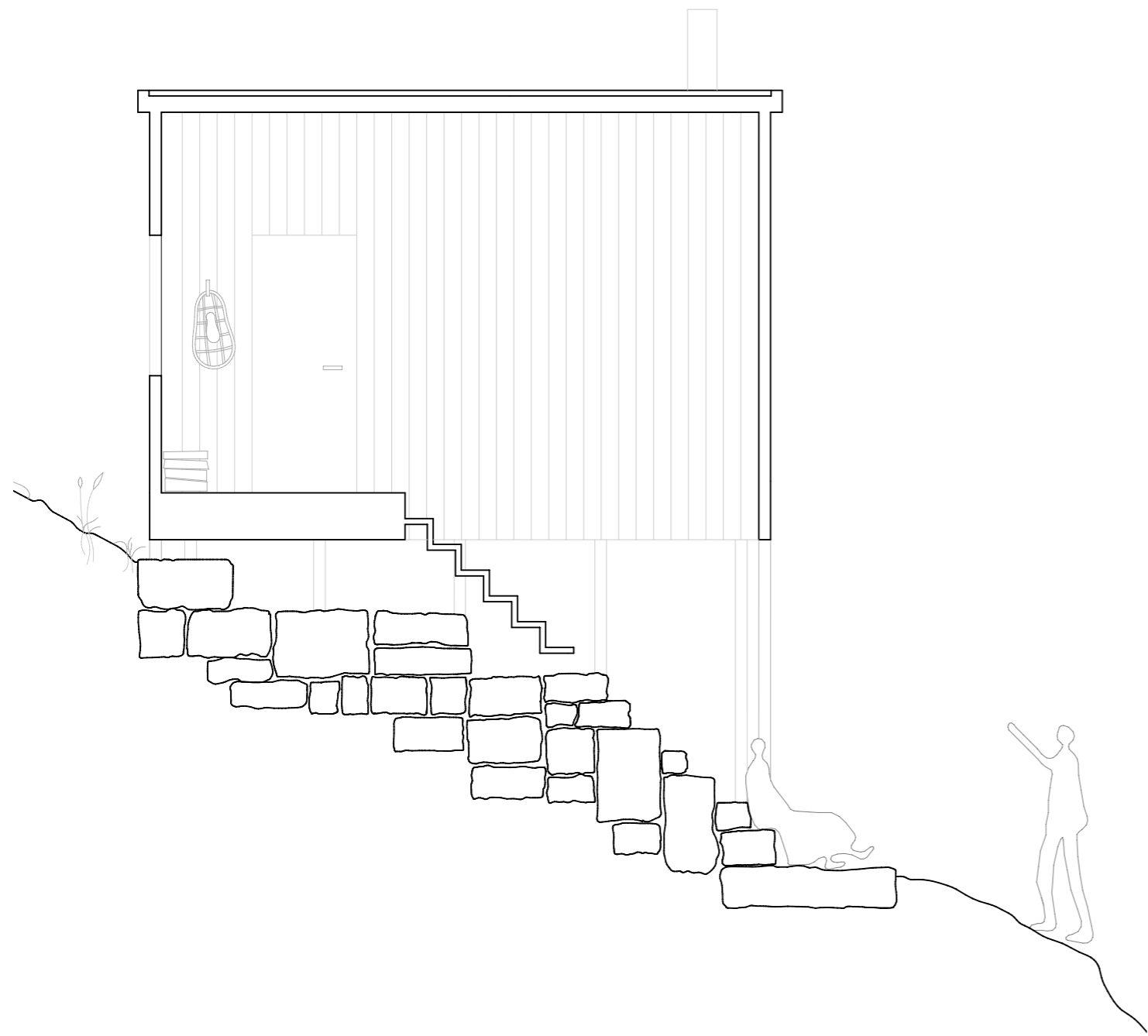
Snitt uu'
