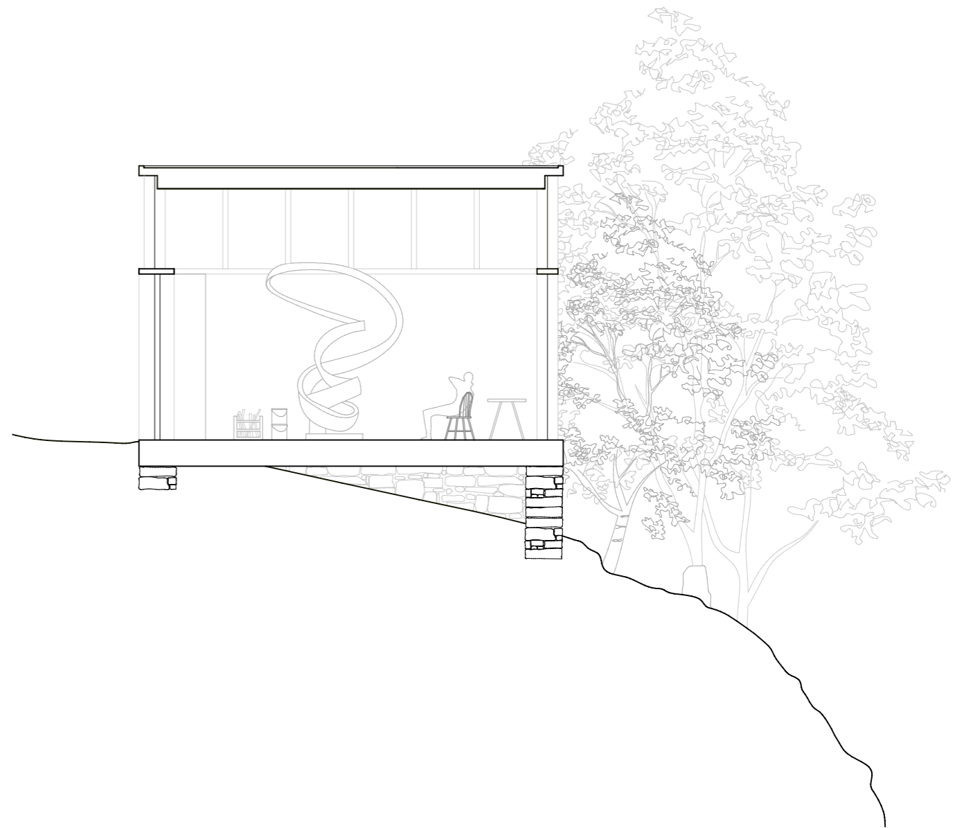
Snitt hh'
