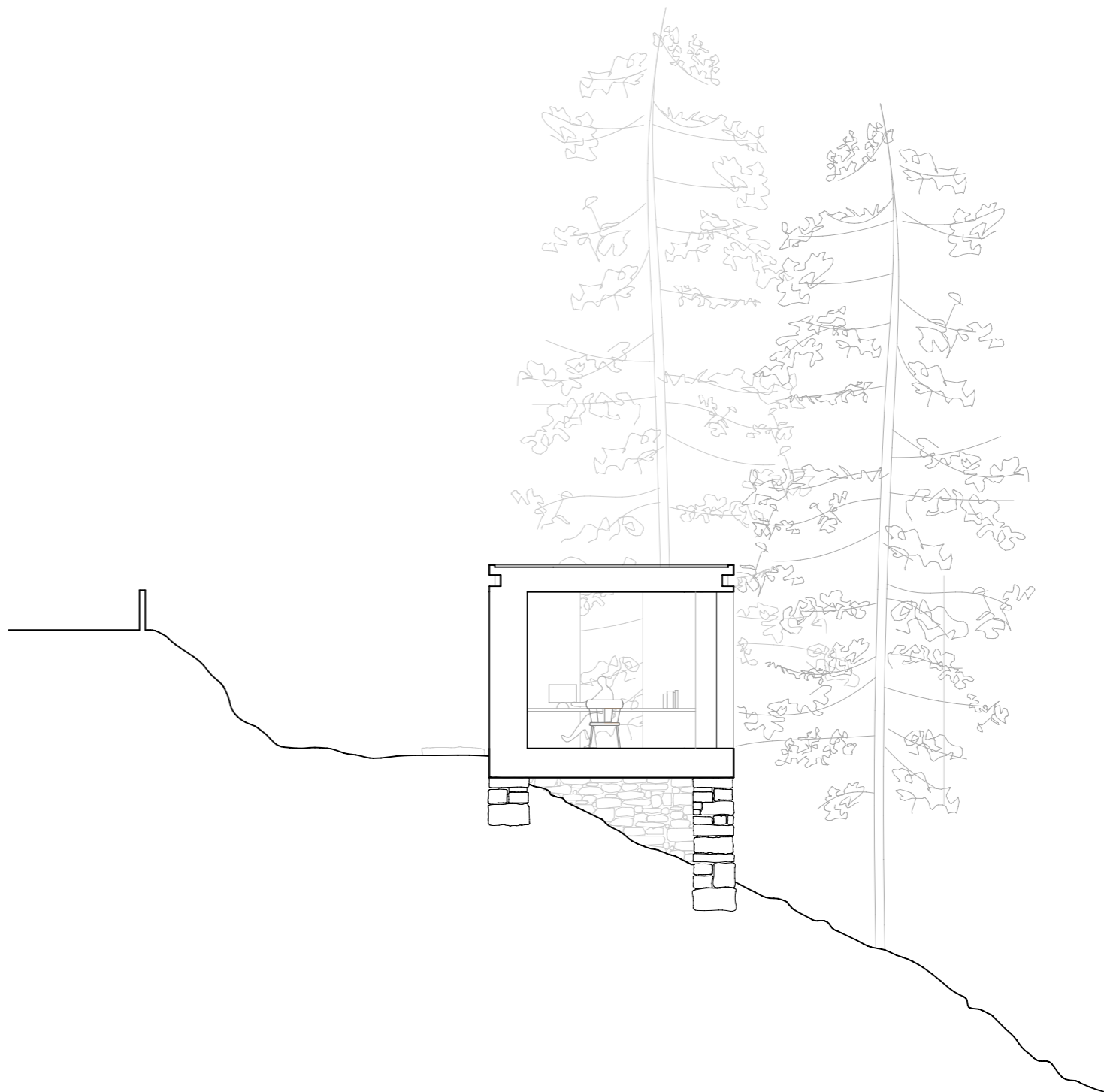
Snitt j-j''
