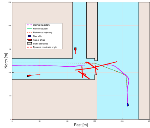
(d) Obstacles activate, breaking the optimal trajectory.
