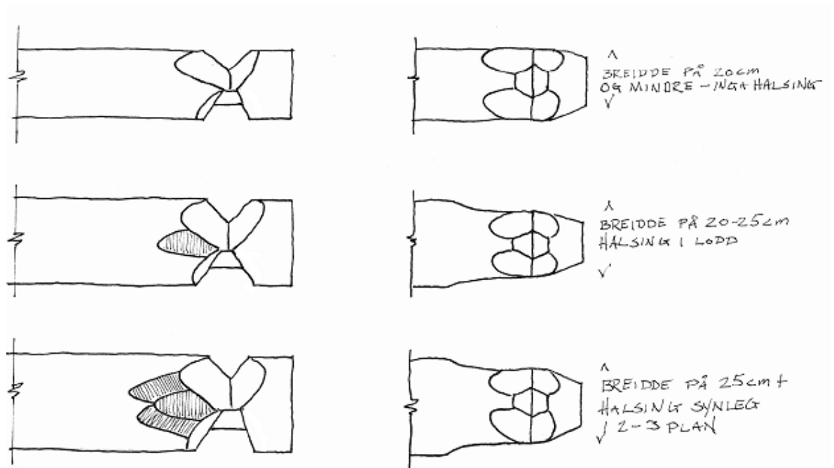
18. Ulike måtar å halse på. Til venstre ser ein laftestokken frå sida. Til høgre ser ein laftestokkane ovanfrå. (Skisse: Aabol)
