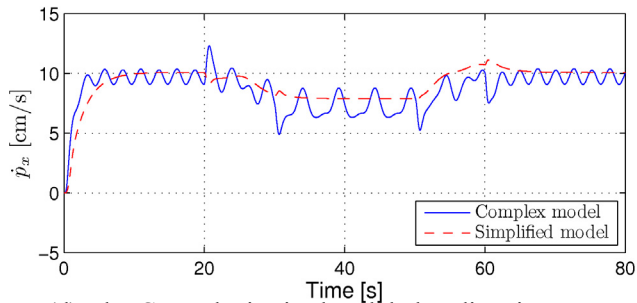
(d) The CM velocity in the global x direction, \dot{p}_x .
