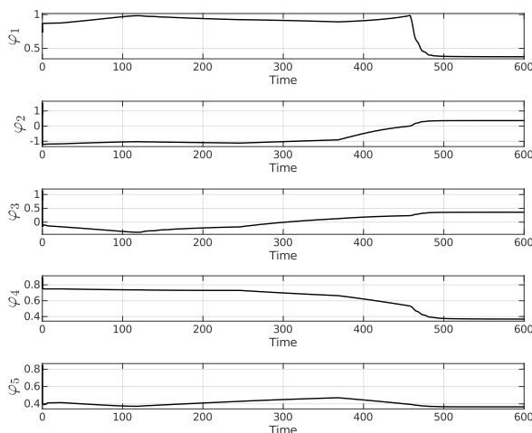
Fig. 6. Dither phases.
