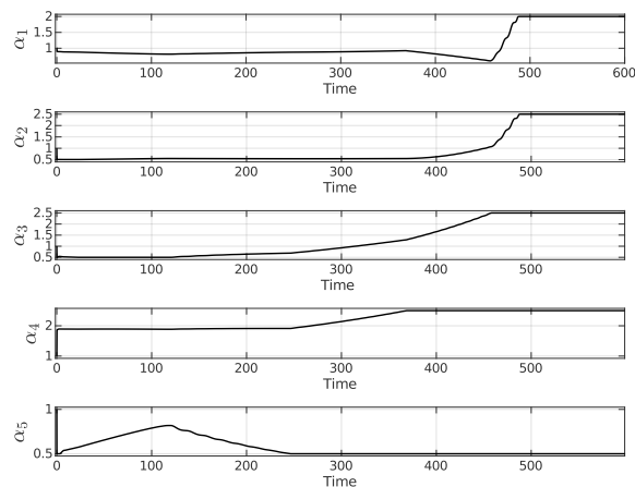
Fig. 5. Dither amplitudes.
