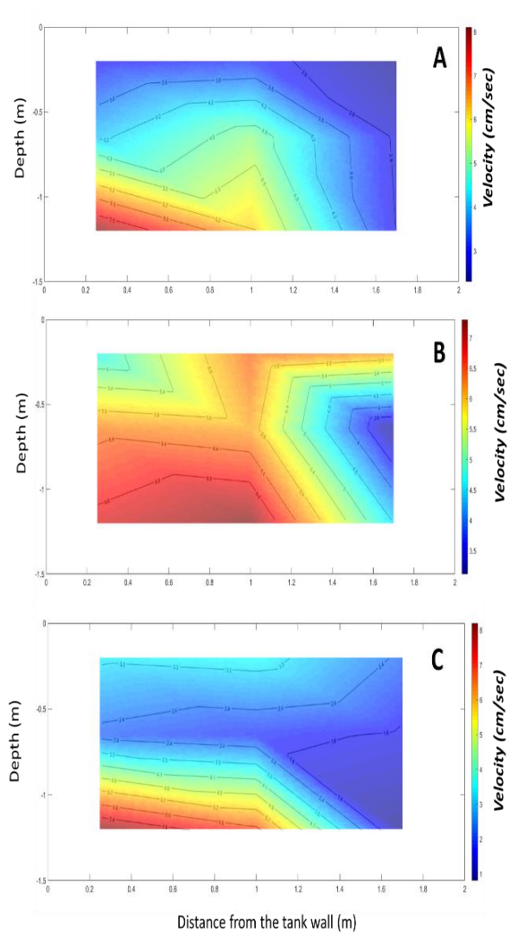
Figur 6 Hastighetsprofiler for kar med volum 20 \text{ m}^3 : A) 201, B)202; C)205. Lavest hastighet er vist i blått, og høyest i rødt. Merk at hastighetskalaen kan være forskjellig på figurene.
