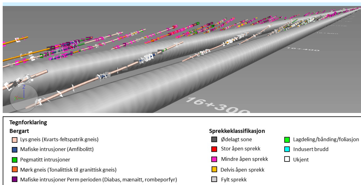
Figur 7.29: Utførte OTV-inspeksjoner langs tunneltraseen for sørlige del av prosjektet. Bildet er laget i NavisWorks.
