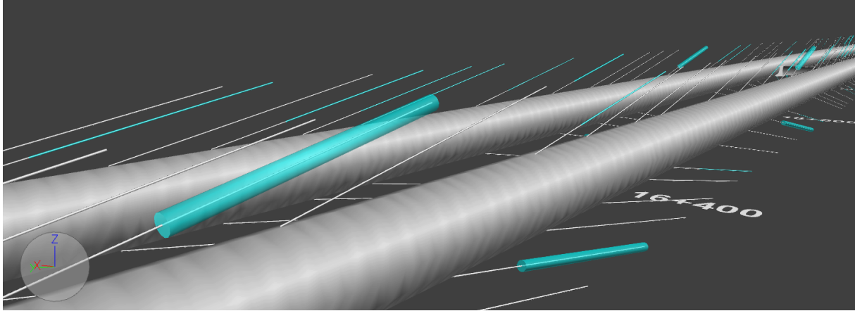
Figur 7.27: Sonderhull langs tunneløpet. De lysblå transparente sylindere representerer vann, hvor tykkelsen varierer ut fra mengde målt vann. Bildet er laget i NavisWorks.
