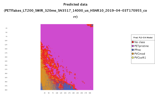
(d) Prediction on dry PET flakes
