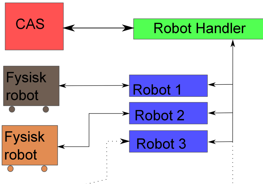
Figur 3.1: Struktur på systemet med et grensesnitt mot robotene. Robotene er ment som alternativer. Det er ikke mulig å oppere mer enn én robot av gangen med nåværende programvare.
