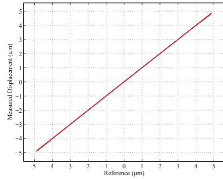
(d) Reference-to-displacement map when using hysteresis compensation.
