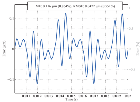
(d) Steady-state measured error \varepsilon .
