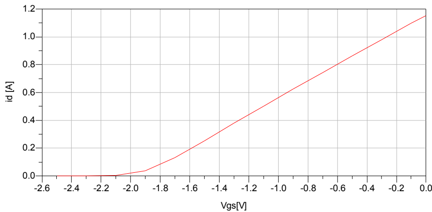
Figur 5.3 Transistorens overføringskarakteristikk.
