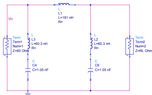
Figur 5.24 Krets for beregning av respons.
