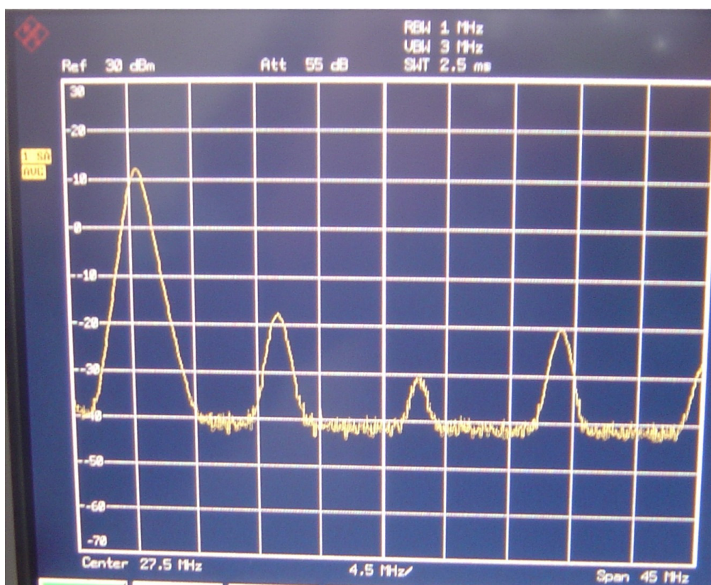
Figur C32 Effektspektrum ved 20dBm inngangseffekt, med \pi -nettverk.
