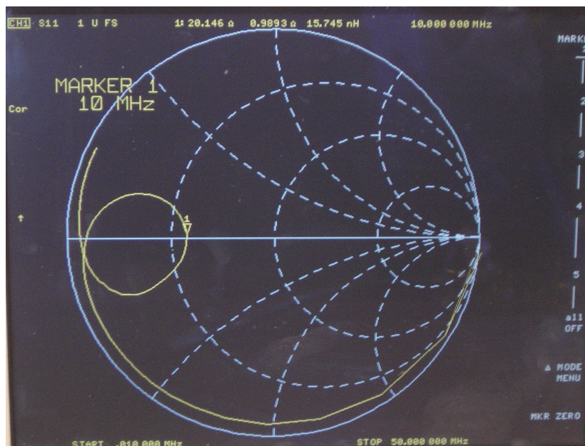
Figur C3 Målt S11 sett inn på \pi -nettverket
