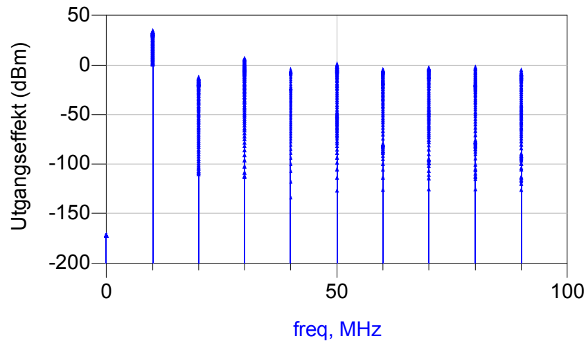
Figur 5.49 Simulert effektspektrum til Dohertyforsterker.
