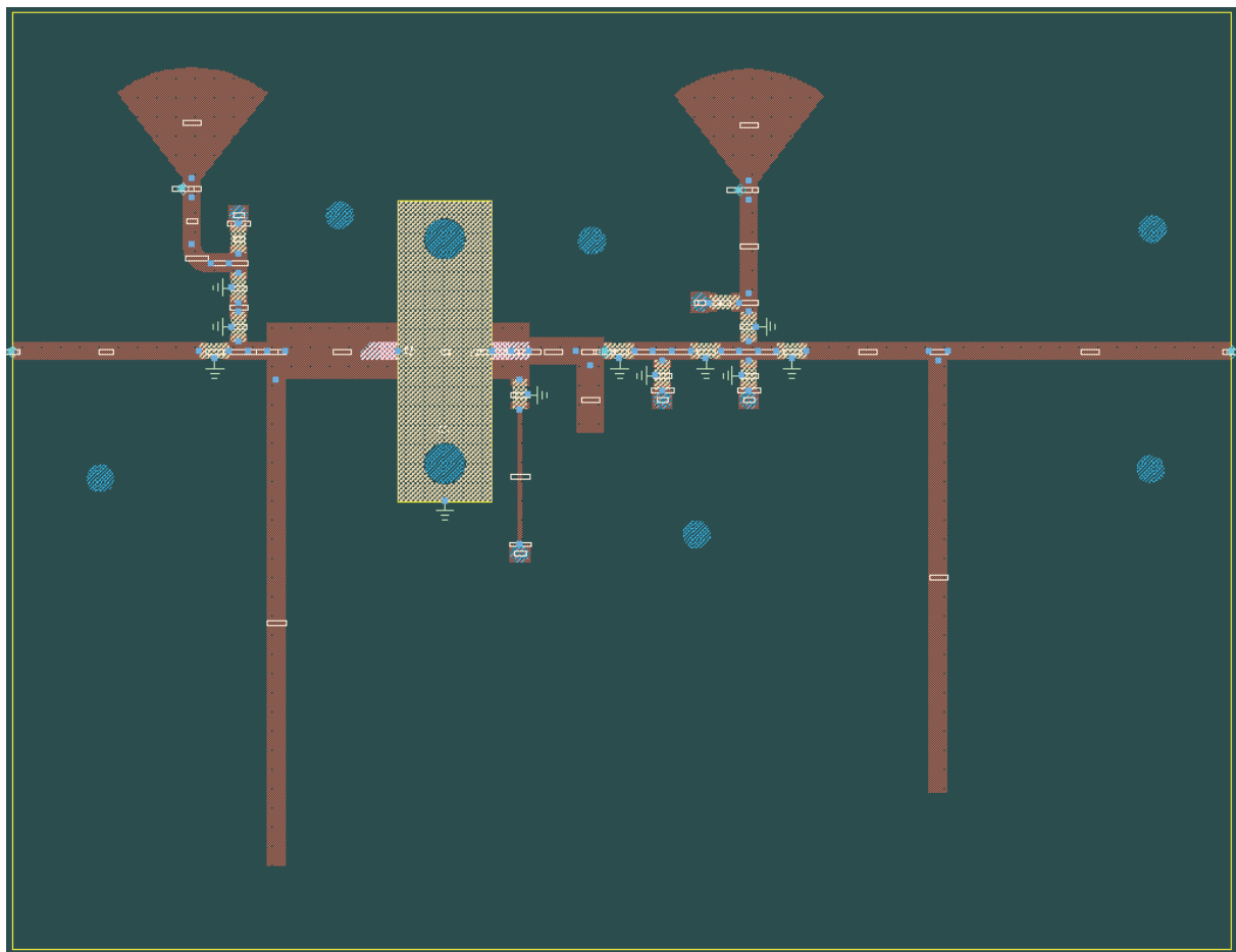
Figur v 6 Kretskortutlegg til klasse F effektförsterker
