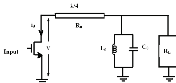
Figur 6 Prinsippskisse av klasse F design med kvartbølgeresonator
