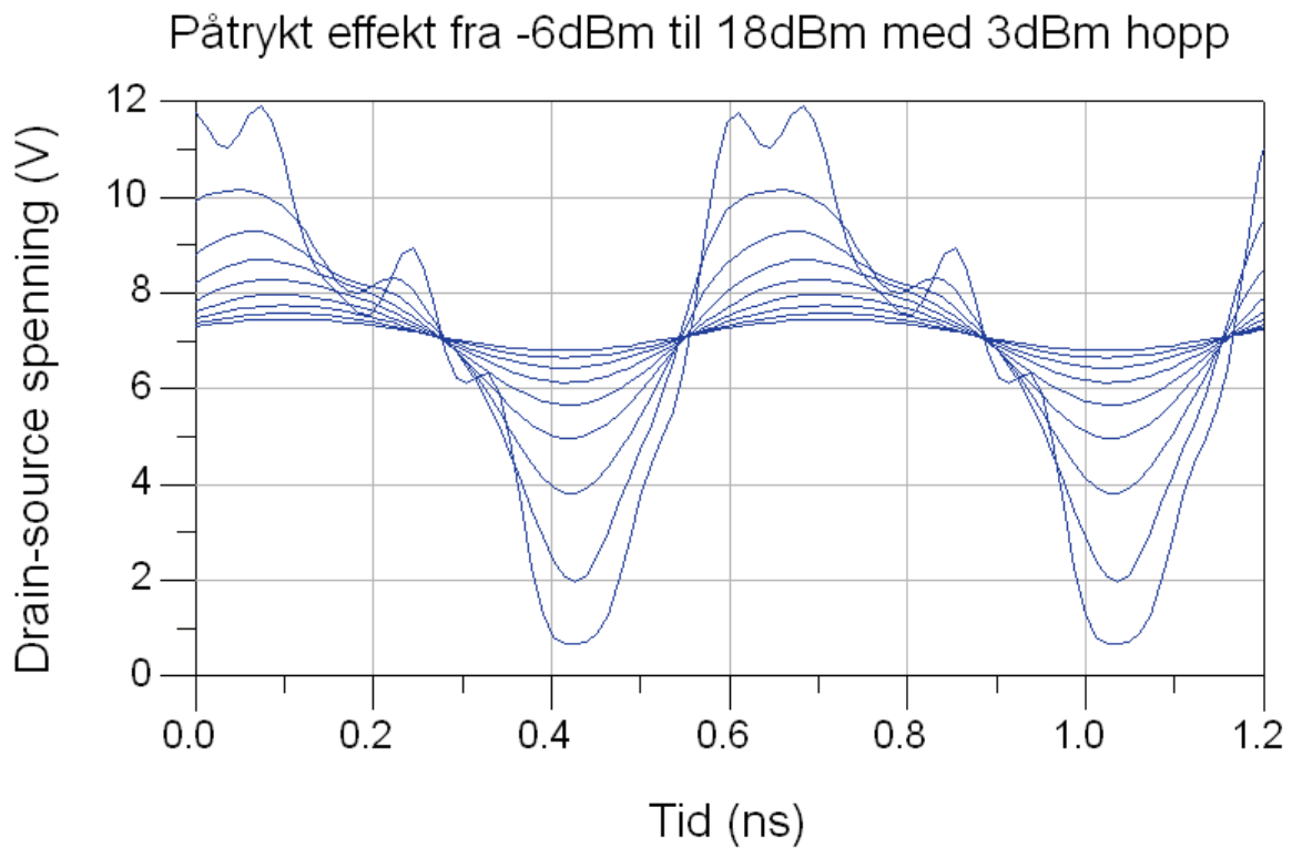
Figur v 22 Simulert drain-source spenning til klasse F effektförsterker
