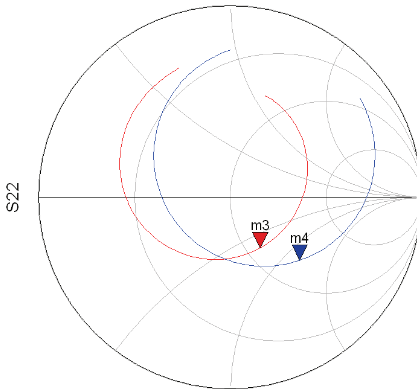
Figur v 27 Målt S_{11} til klasse AB og klasse F effektförsterker
