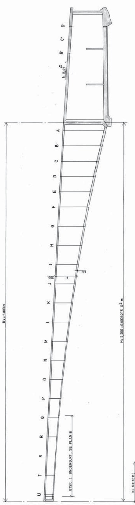
LENGDESNIITT I BRUAKSE 1:200
