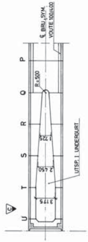
PLAN B, UNDERGURT VED FLUGE 1:200
