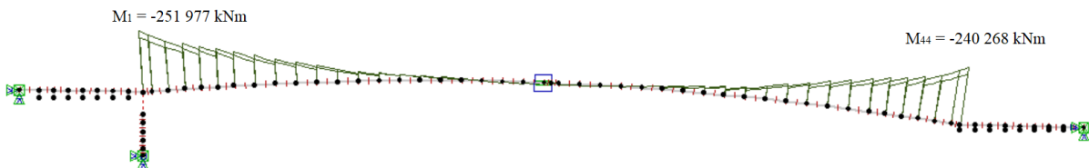
Figur 11.9: Dimensionerende moment SLSb uten trafikk
