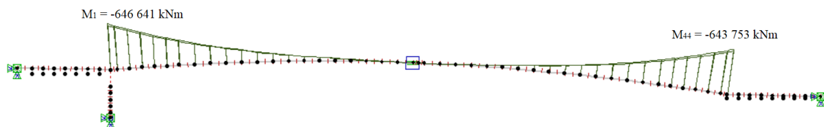
Figur 11.10: Dimensionerende moment SLSb uten forspenning og trafikk
