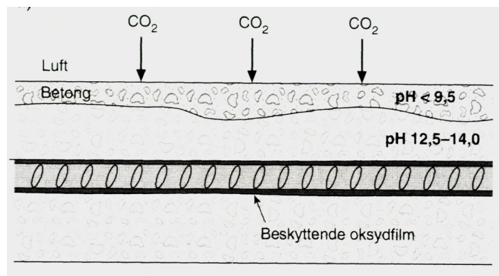
Figur 4.2: Karbonatisering [7]
