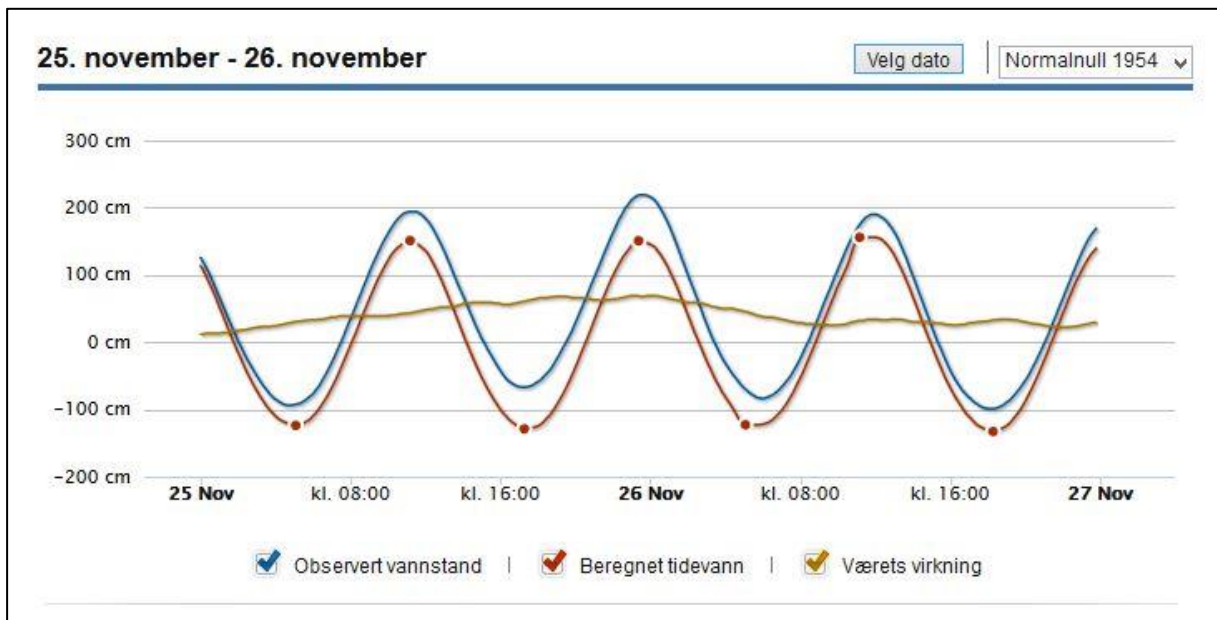
Figur 4-5 Vannstand i Trondheim den 25-26. november 2011 under stormen Berit.
