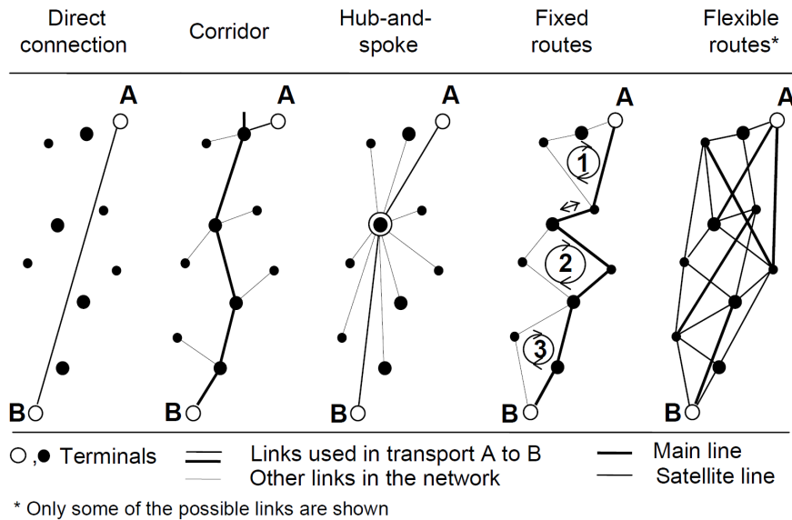
Figur 2.4: Grafisk fremstilling av mulige terminalstrukturer [38]
