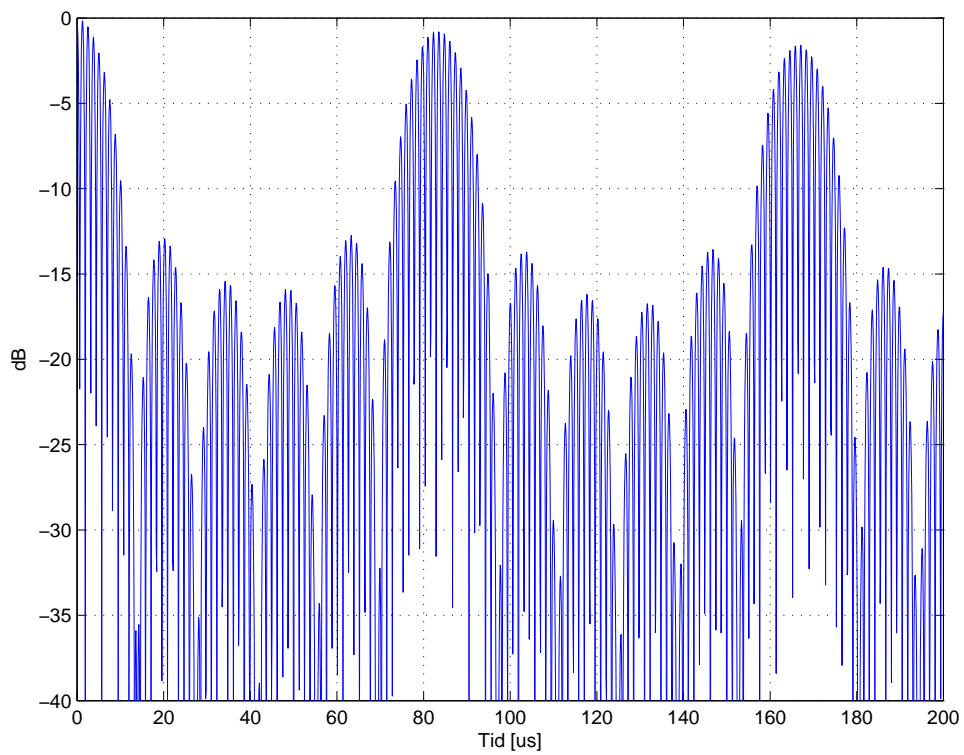
Figur 8: Tidsoppløsning for kampsuls
