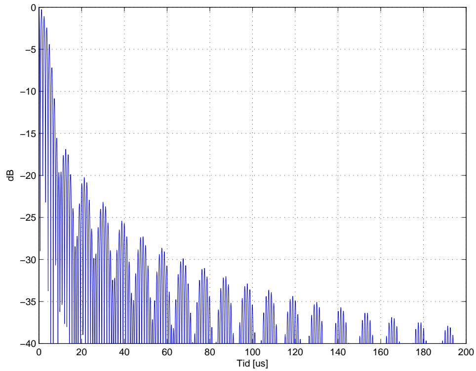
Figur 7: Tidsoppløsning for lineært chirp
