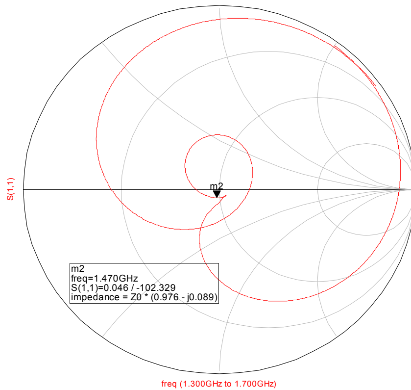
Fig. C.14 Impedanstilpasning Prototyp II ved v_r = 29V
