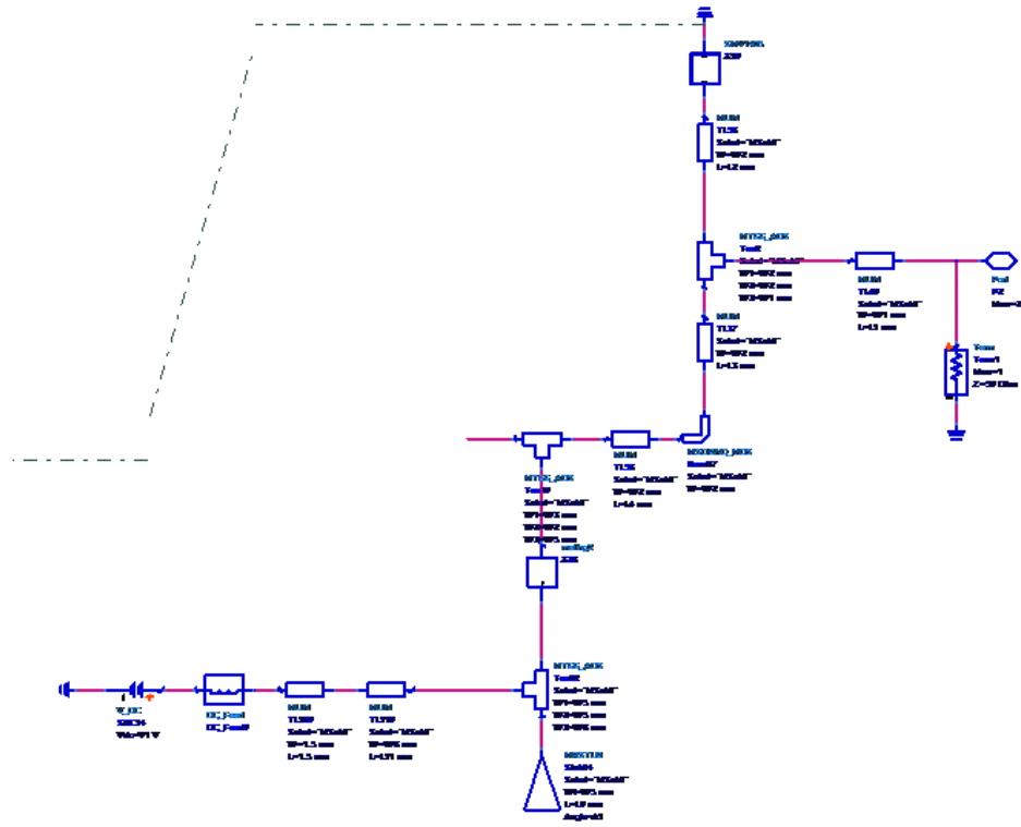
Skjemategning 9 Prototyp II del 5
