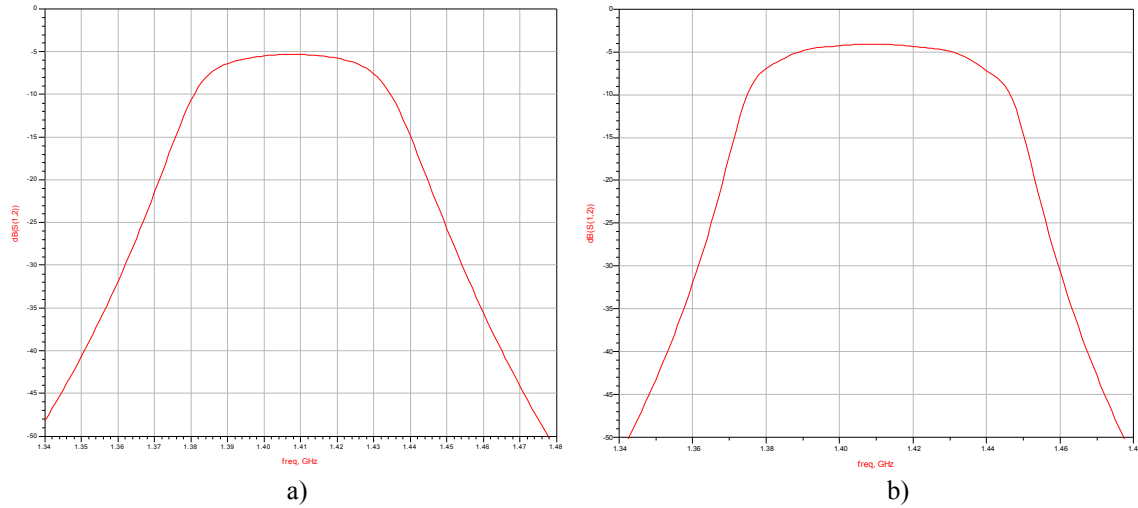
Figur 6.9 Filterkarakteristikk for sjettede ordens filter etter optimalisering. a) ujusterbart filter, b) med kondensatorer på resonatorendene.
