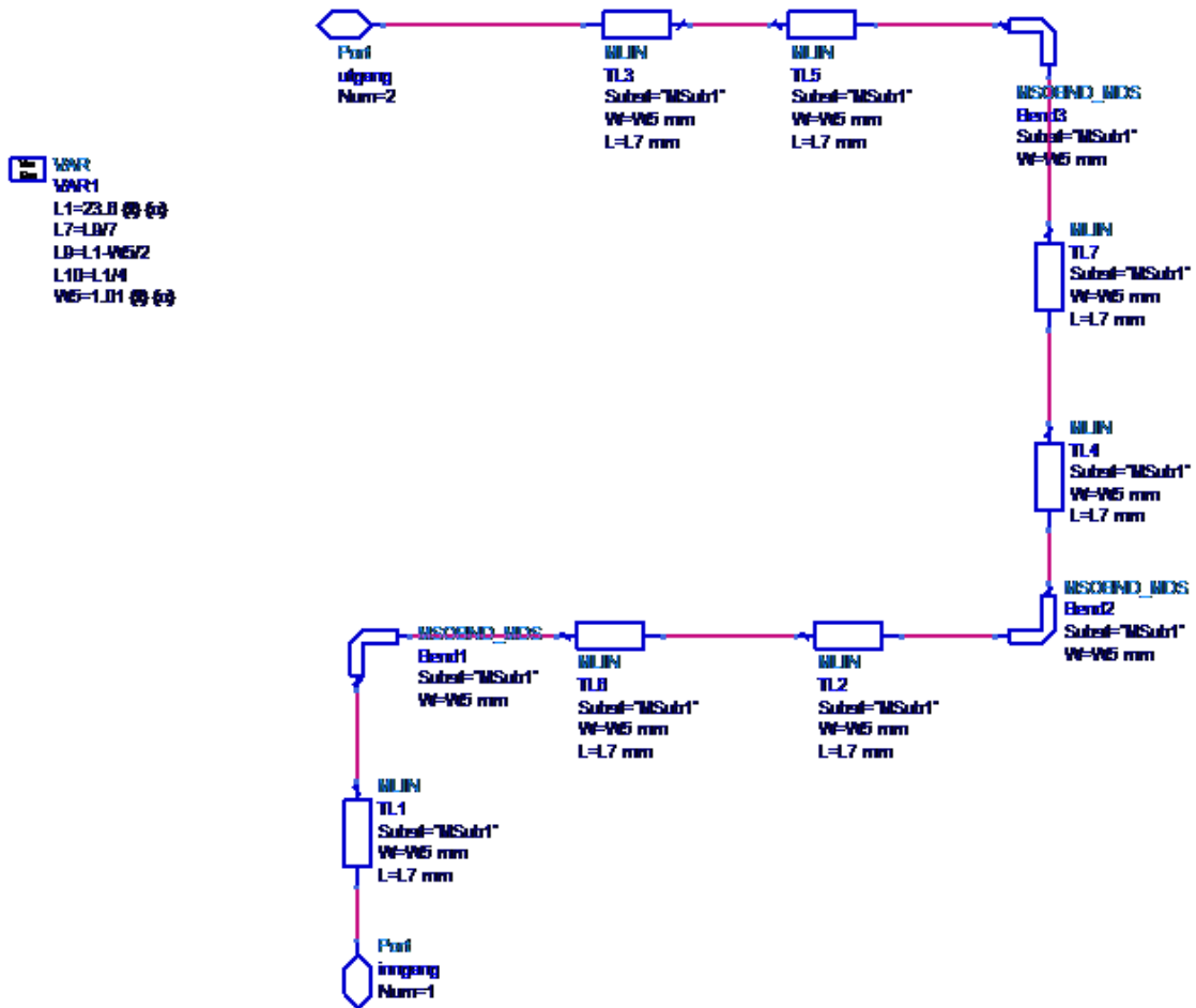
Skjemategning 11 Matenetverk 2 til Prototyp II
