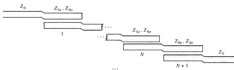
Figur 5.2 Utlegg av parallellkoblet resonator-filter. (Hentet fra [3])
