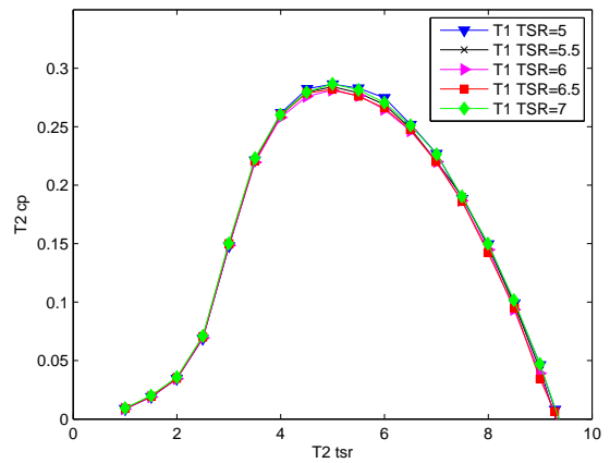
(d) T2 POWER PERFORMANCES: 9D distance, high background turbulence
