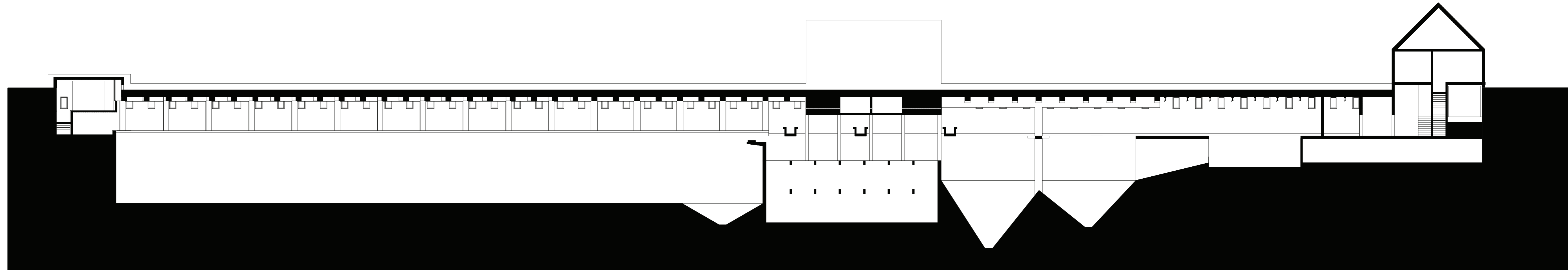
SNITT AA 1:200
