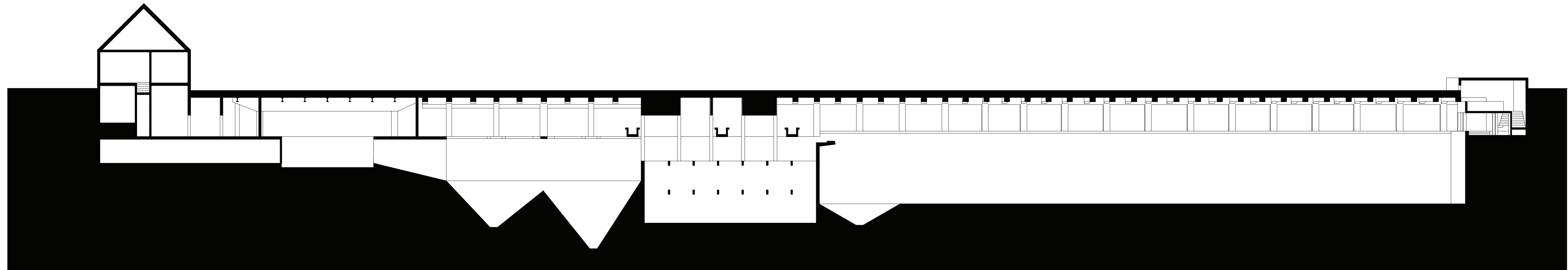
SNITT BB 1:200
