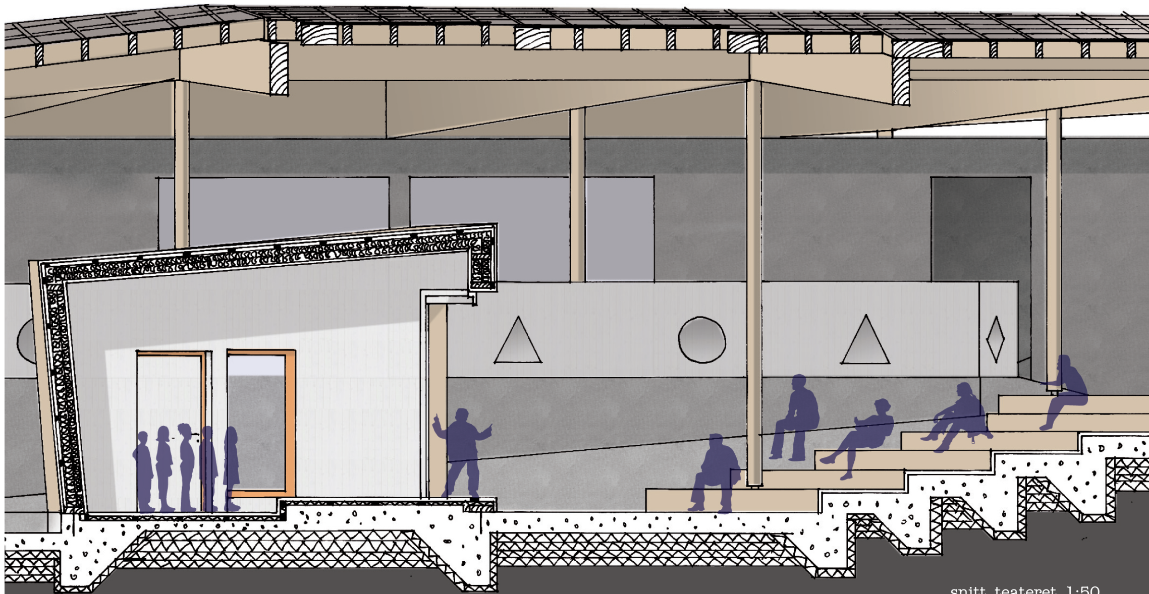
snitt, teateret 1:50
