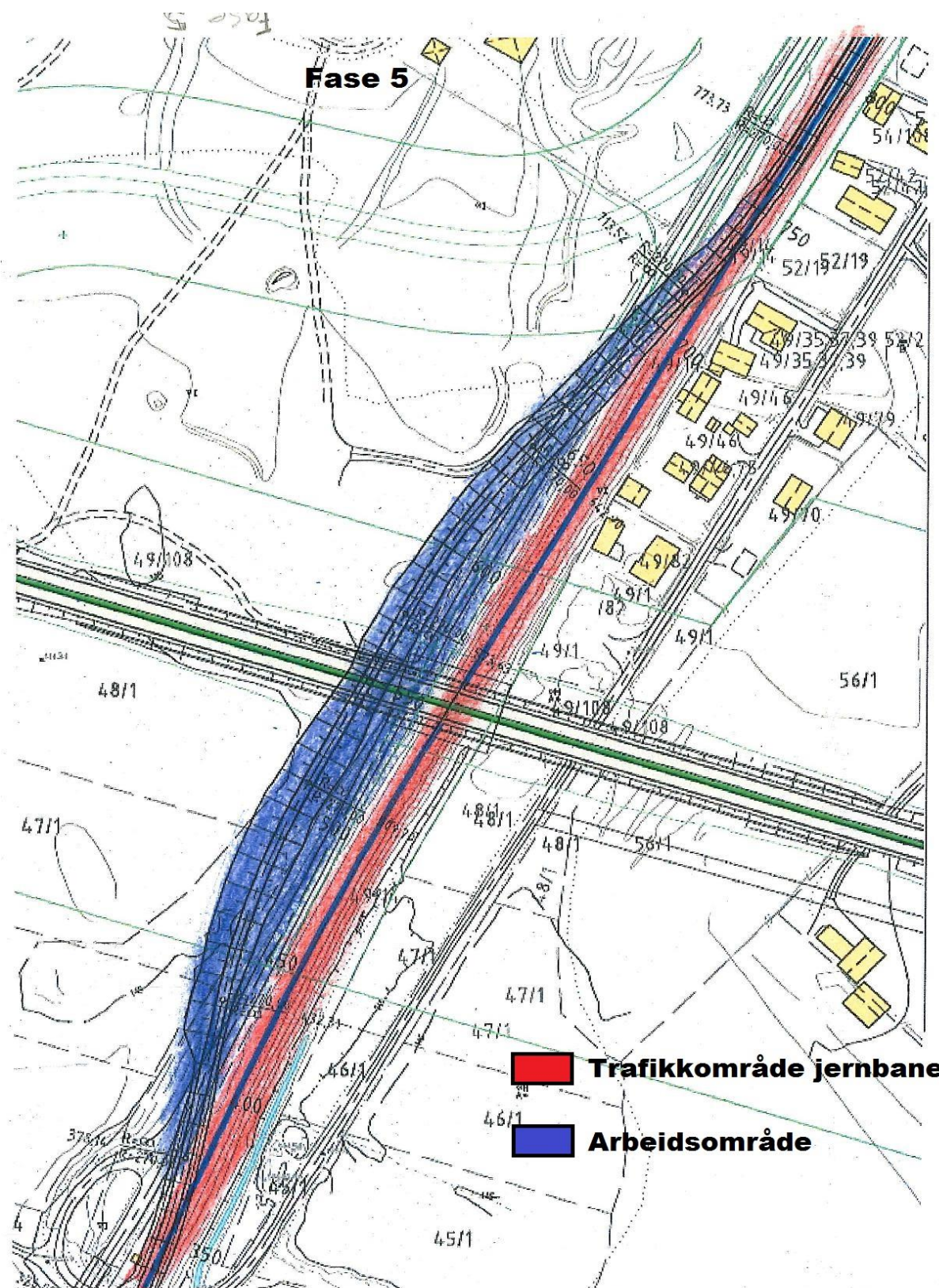
Fase 5: Interimsporet med fylling fjernes.
