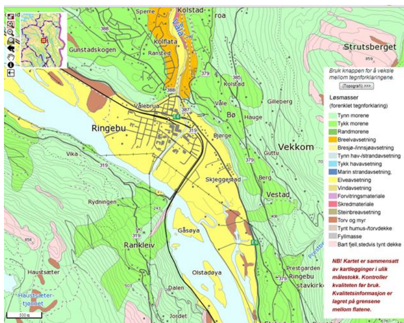
Figur 7: Løsmassekart, Ringebu, http://geo.ngu.no/kart/losmasse/ 19.02.13
